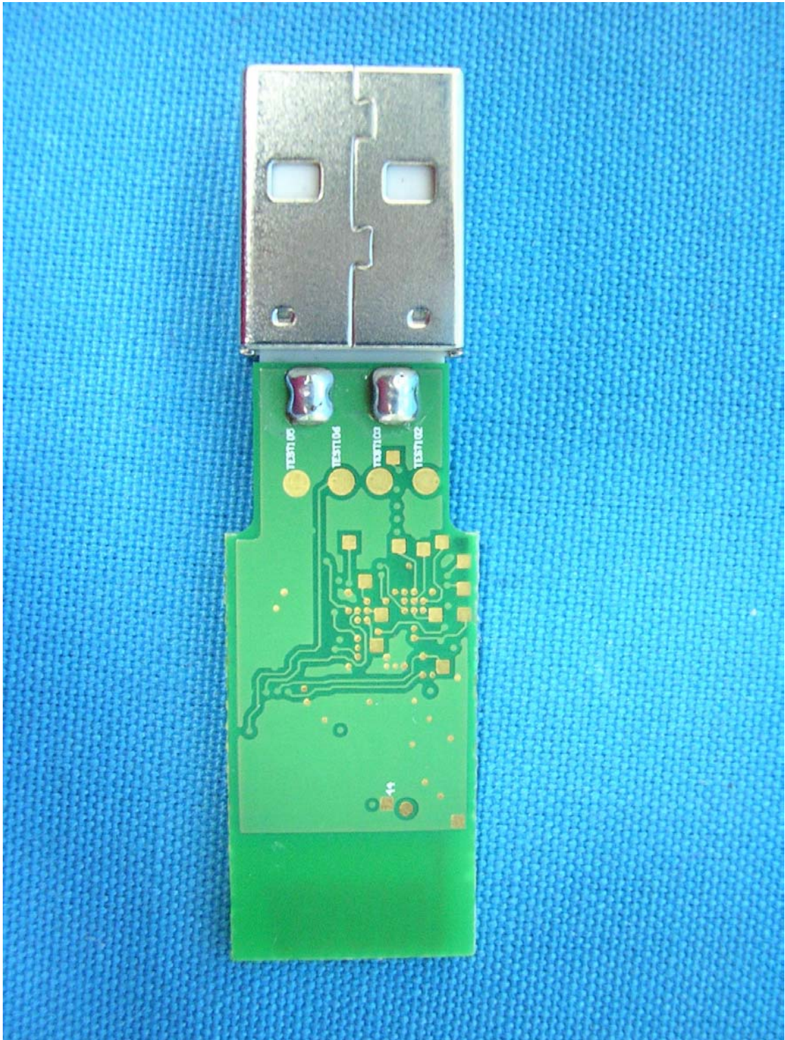
(9) EUT Photo
