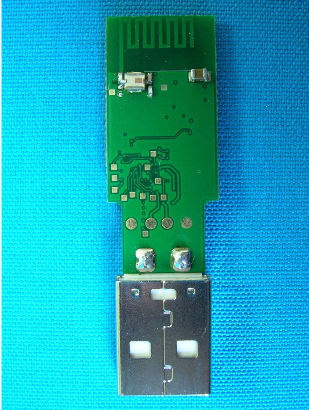
(5) EUT Photo
