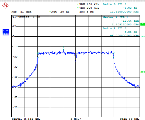
802.11n(HT20)
