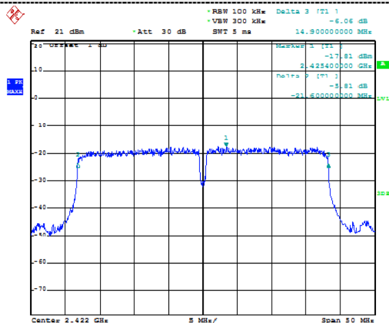
802.11n(HT40)
