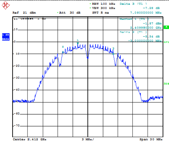
802.11b
