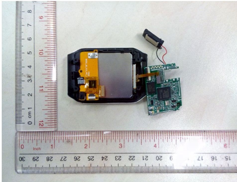
(3) EUT Photo
