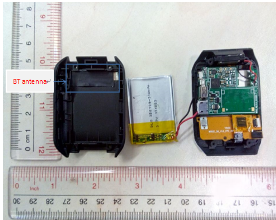
(2) EUT Photo
