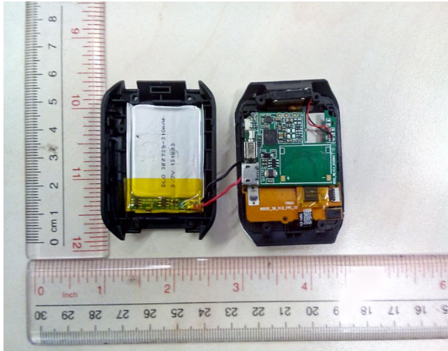
(2) EUT Photo
