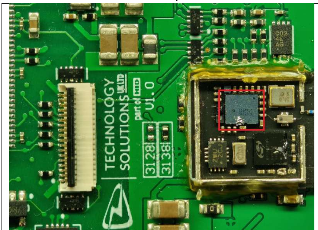
BLE Chip
