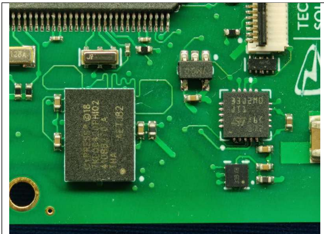
BLE Chip
