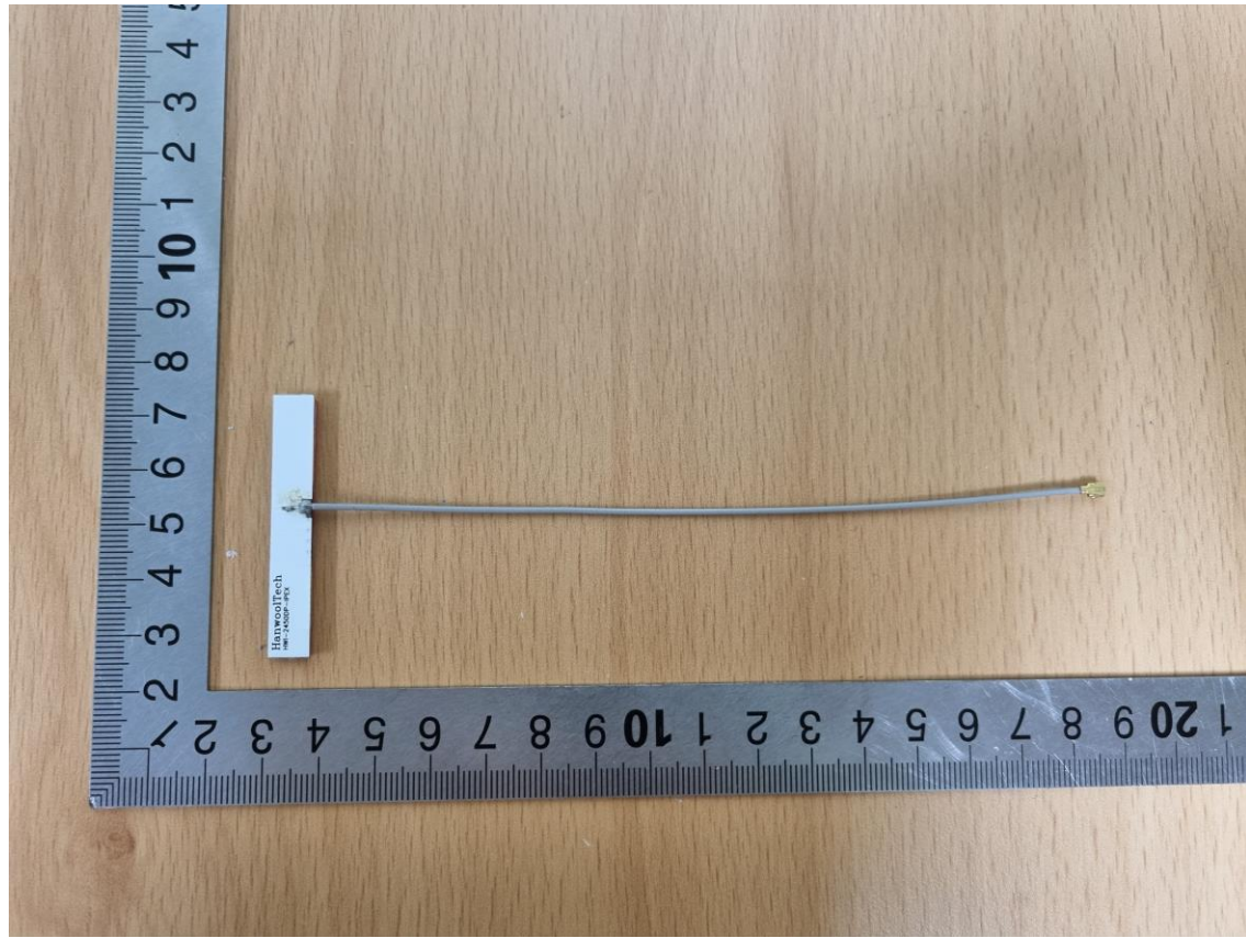
PCB Antenna (HWI-2450DP-IPEX-150 _ 2.248 dBi)
