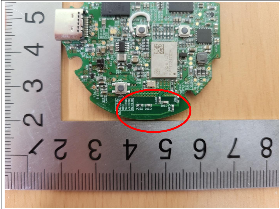
BT&WLAN Antenna
