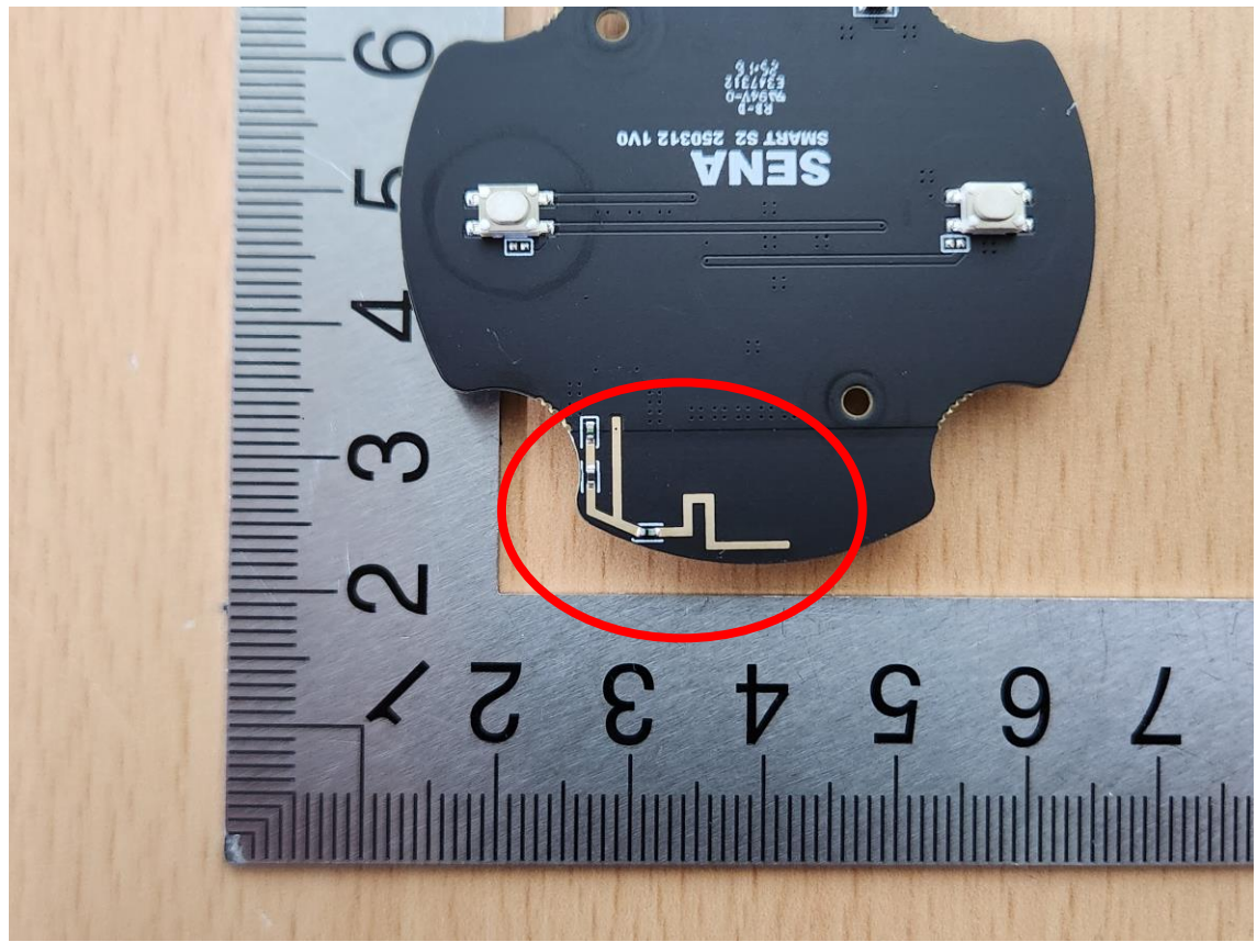
MESH Antenna 2 (M/N: LATITUDU S2 SUB)
