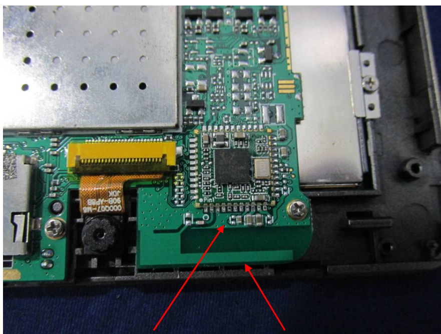
WIFI&BT Module
