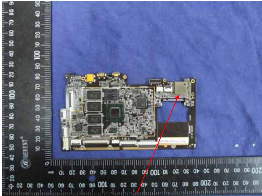
WIFI+BT Module
