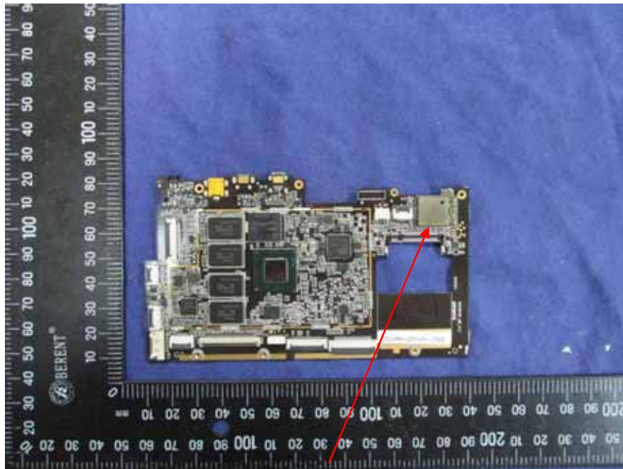
WIFI+BT Module
