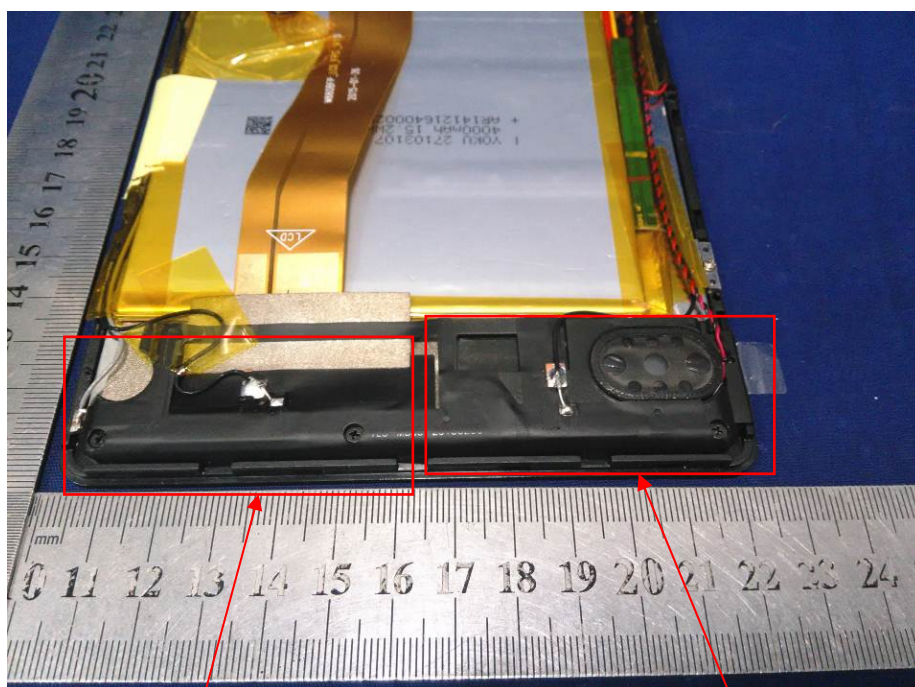
Bluetooth/Wifi Antenna
