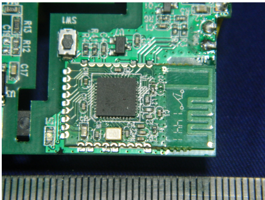
Zigbee Module
