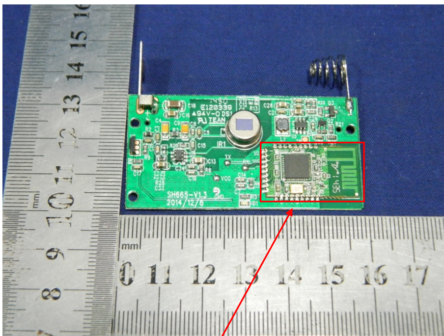
Zigbee Module
