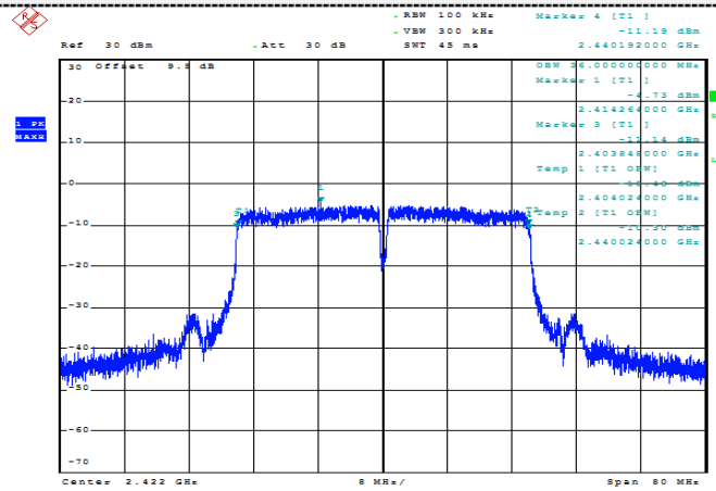
802.11n(HT40)
