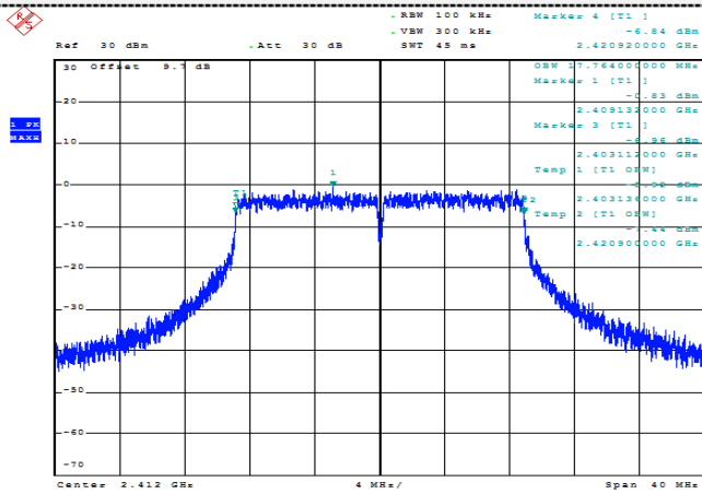
802.11n(HT20)
