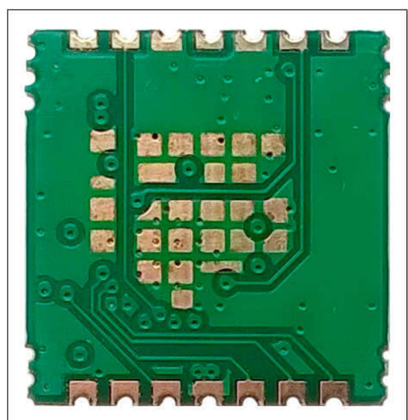
Module BOTTOM
