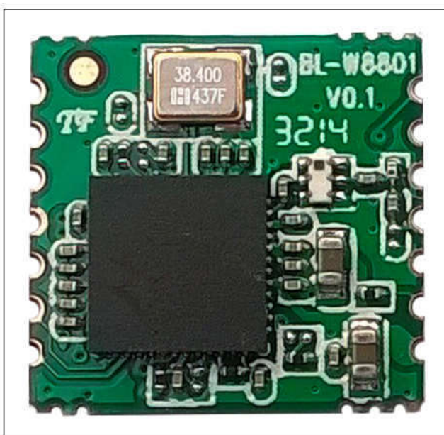
Module TOP
