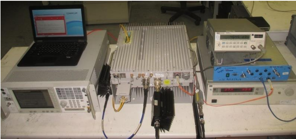
Tx2 output
