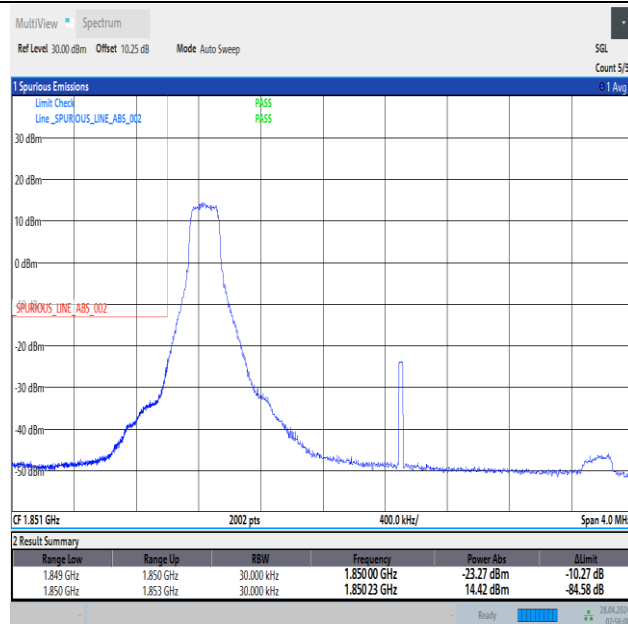
Band2_3MHz_QPSK_18615_1RB#0
