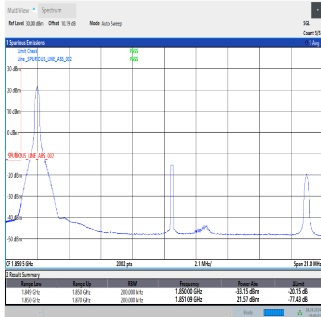
Band2_20MHz_QPSK_18700_1RB#0
