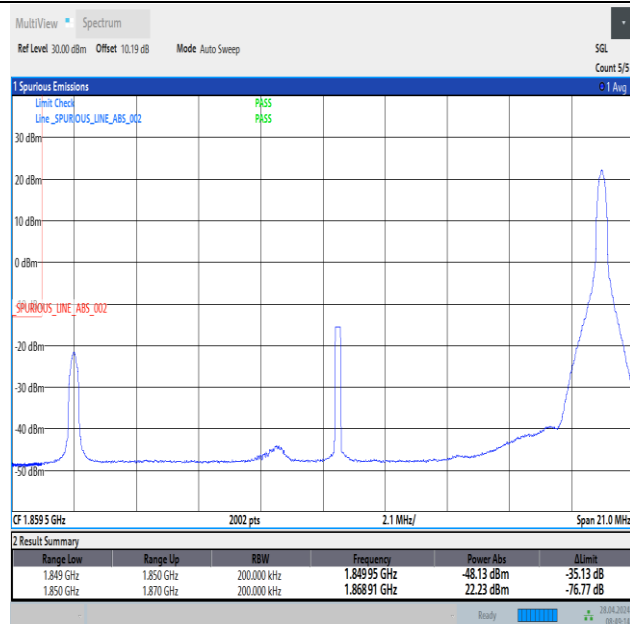
Band2_20MHz_QPSK_18700_1RB#99
