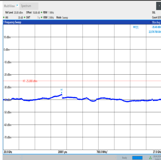
Band41_15MHz_QPSK_39725_75RB#0_20000~27000_20000~27000
