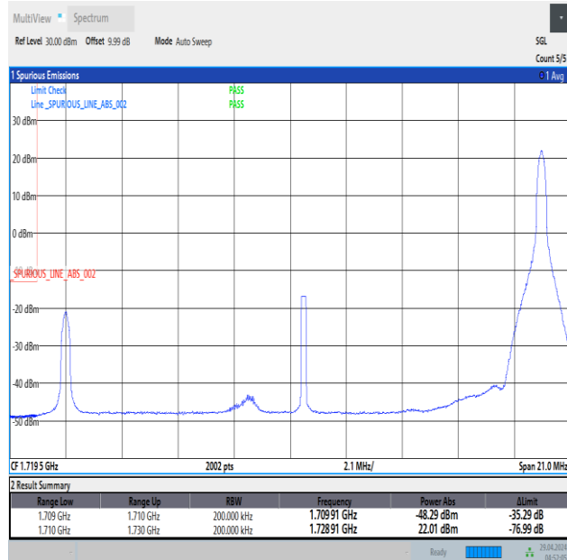
Band66_20MHz_QPSK_132072_1RB#99
