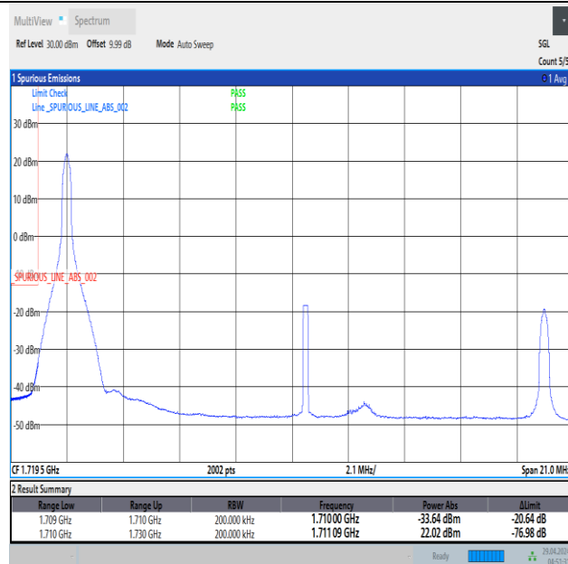
Band66_20MHz_QPSK_132072_1RB#0
