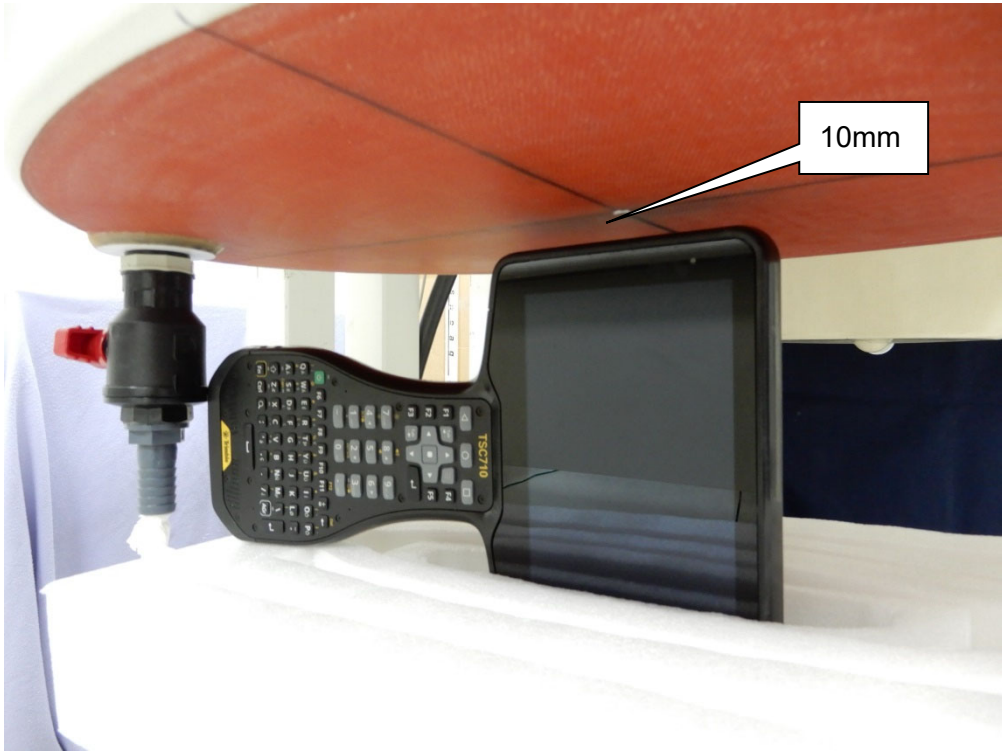
EUT Left-side -10mm (Aux Antenna)
