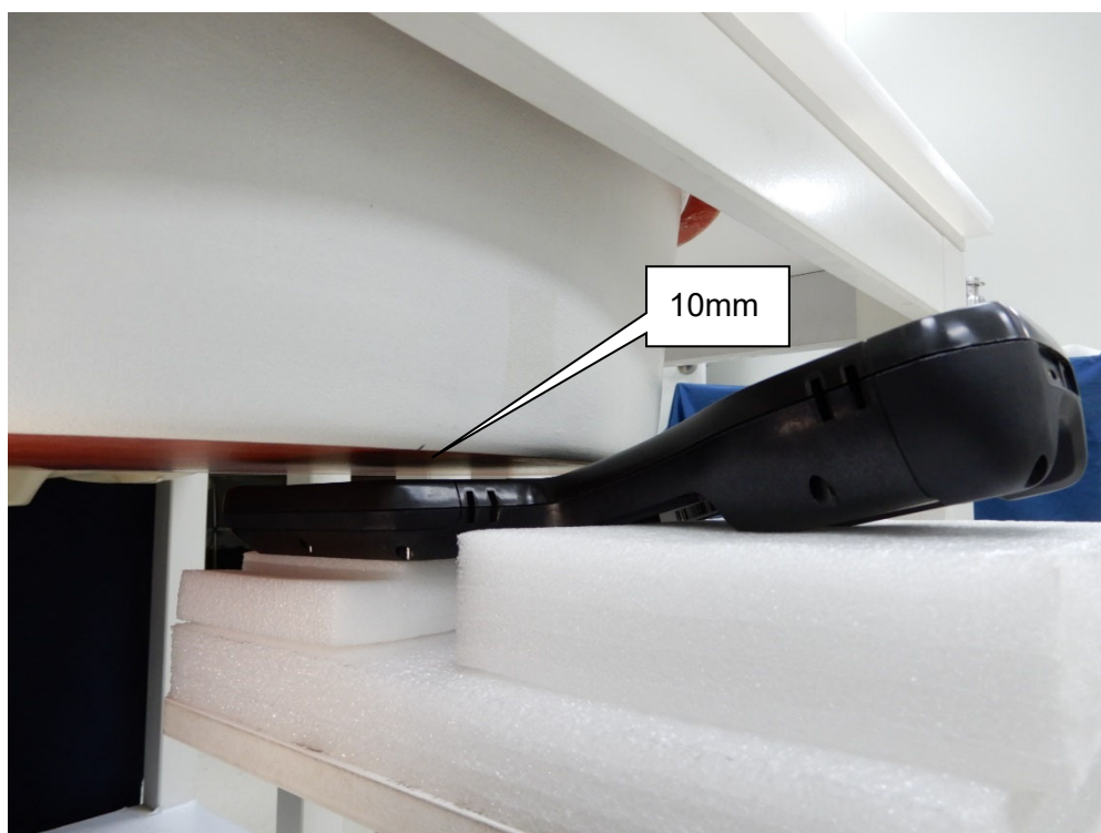
EUT Front - 10mm (Aux Antenna)
