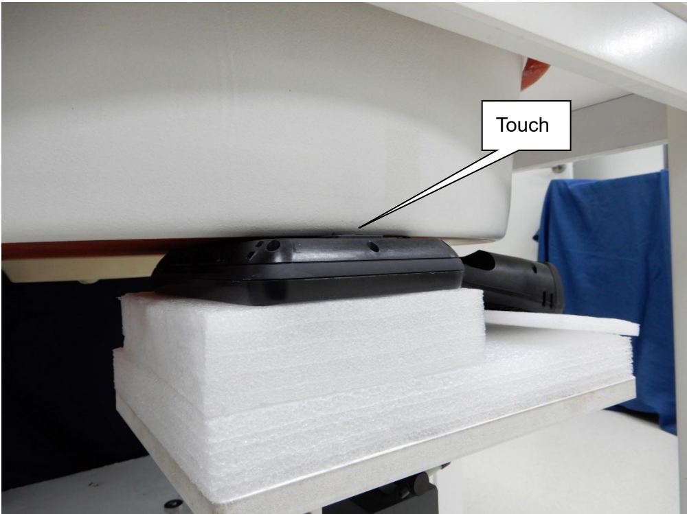
EUT Back - 0mm (Aux Antenna)
