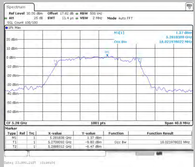
11N20MIMO-Ant2-5280
