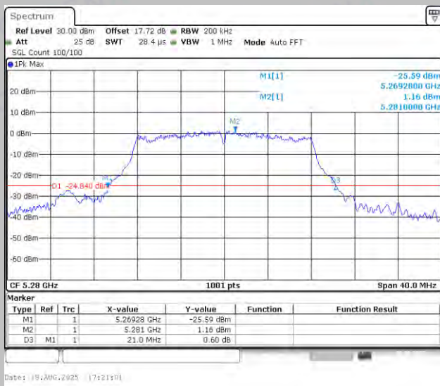
11A-Ant1-5280
