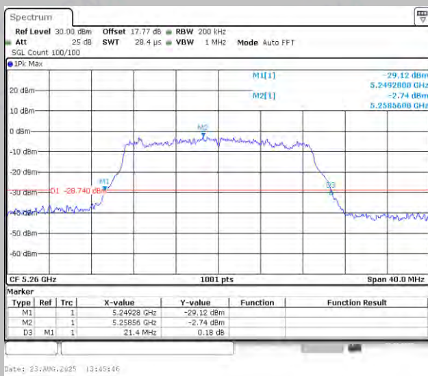
11AC20MIMO-Ant1-5260
