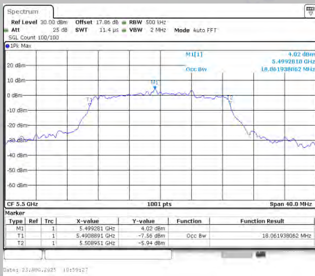
11N20MIMO-Ant1-5500
