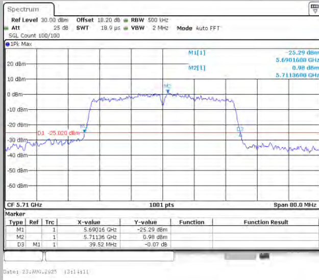
11N40MIMO-Ant1-5710
