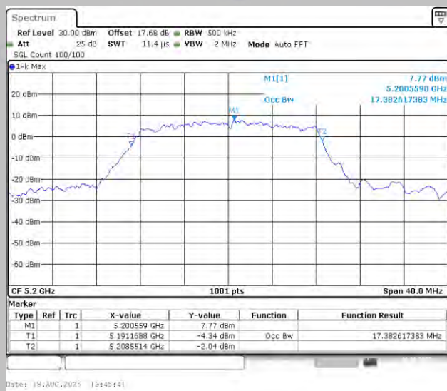
11A-Ant1-5200
