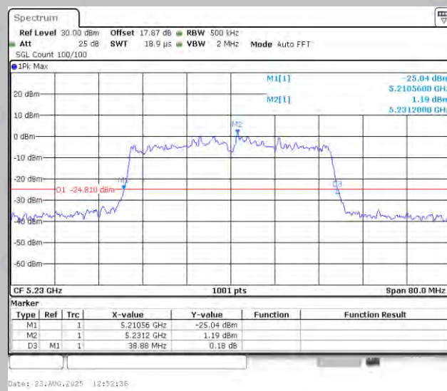
11N40MIMO-Ant2-5230
