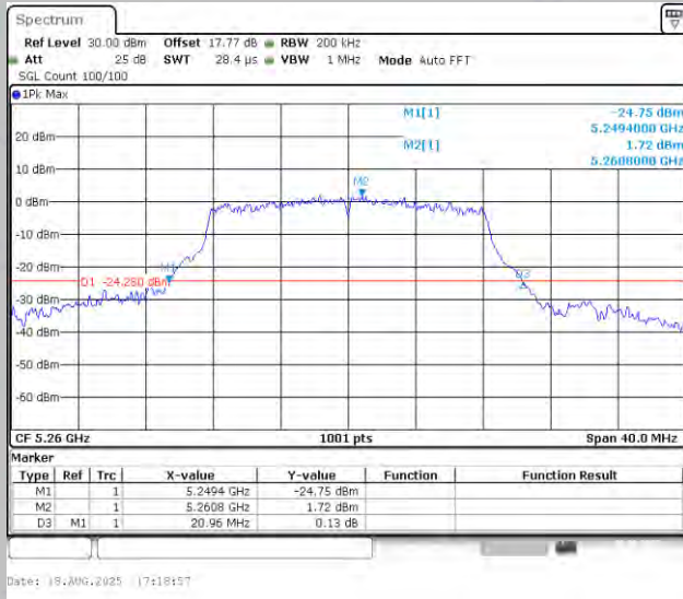
11A-Ant1-5260
