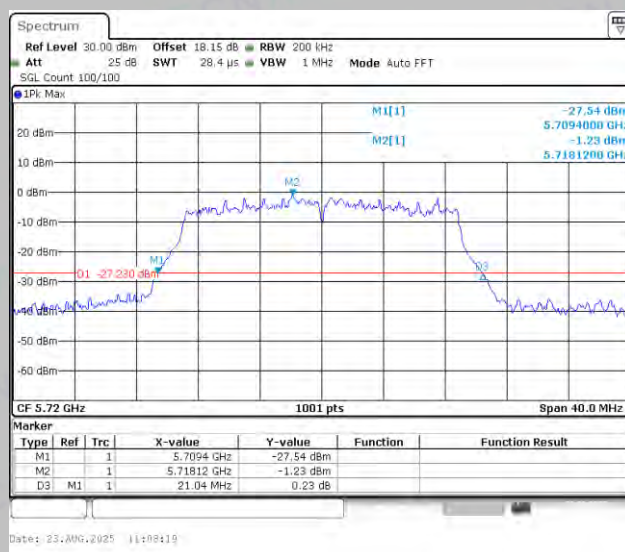
11N20MIMO-Ant2-5720
