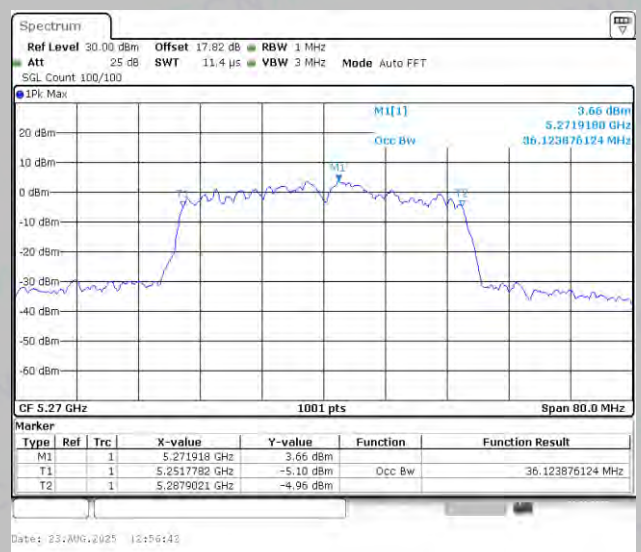
11N40MIMO-Ant2-5270
