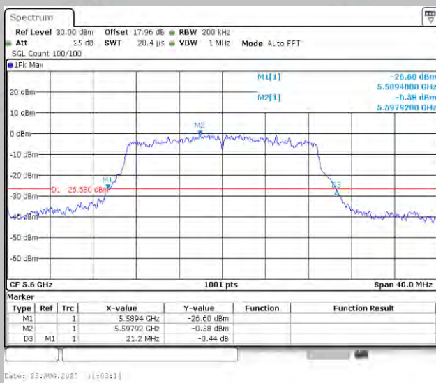
11N20MIMO-Ant1-5600
