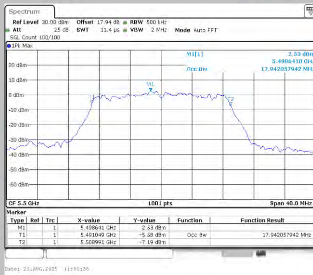
11N20MIMO-Ant2-5500
