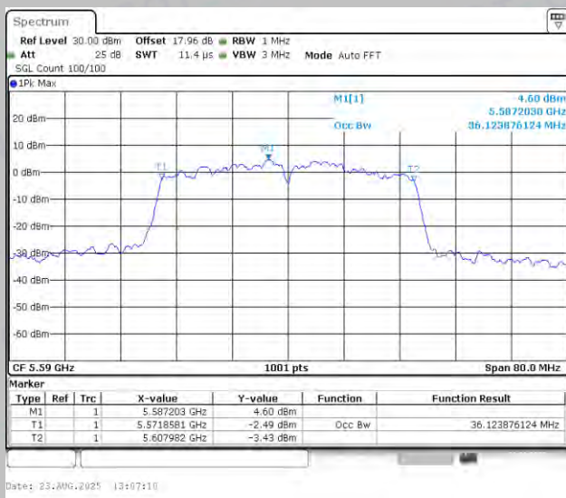
11N40MIMO-Ant1-5590
