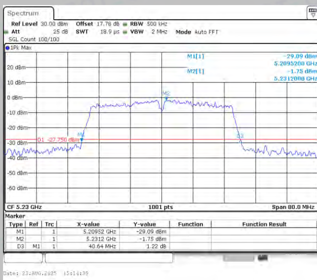
11AC40MIMO-Ant1-5230
