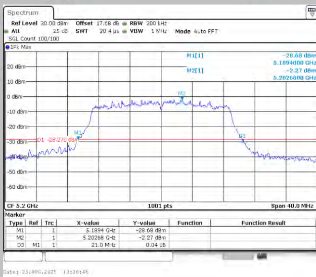
11N20MIMO-Ant1-5200
