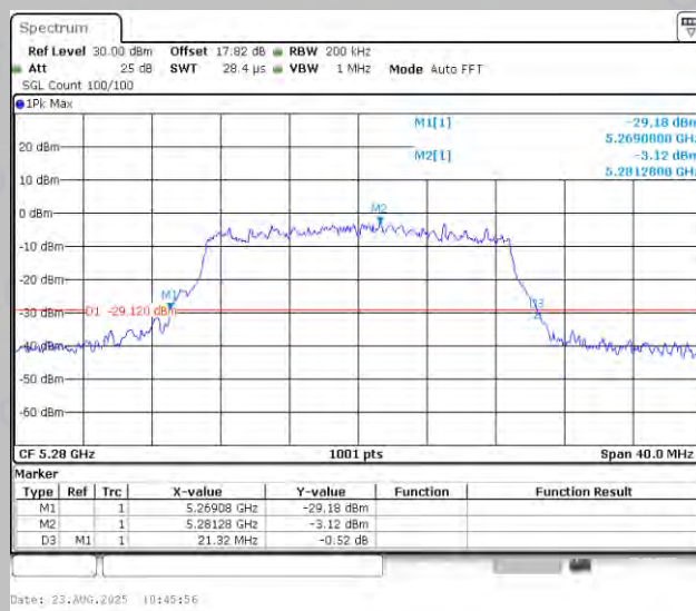
11N20MIMO-Ant2-5280
