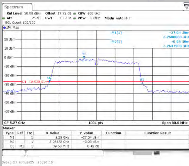
11AC40MIMO-Ant1-5270
