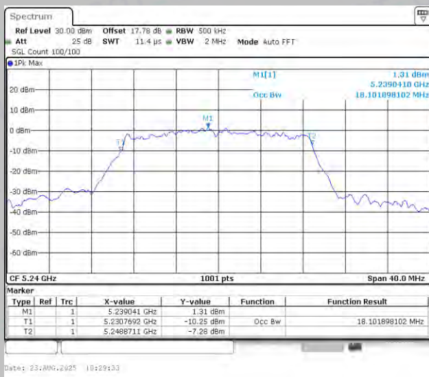
11N20MIMO-Ant1-5240
