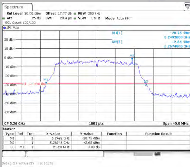
11N20MIMO-Ant1-5260
