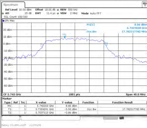
11A-Ant1-5745
