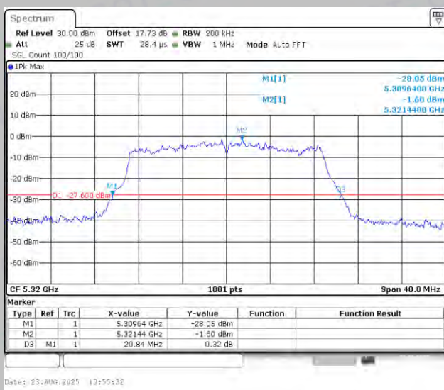
11N20MIMO-Ant1-5320
