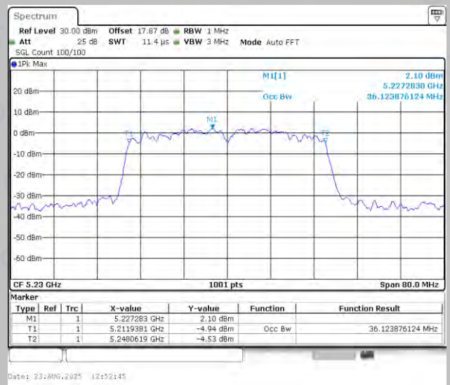
11N40MIMO-Ant2-5230
