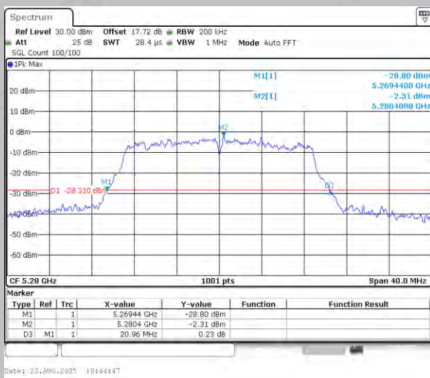
11N20MIMO-Ant1-5280
