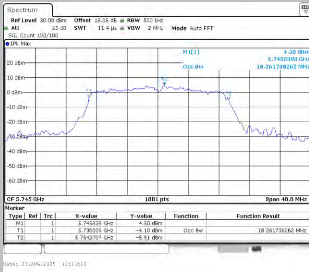
11N20MIMO-Ant1-5745
