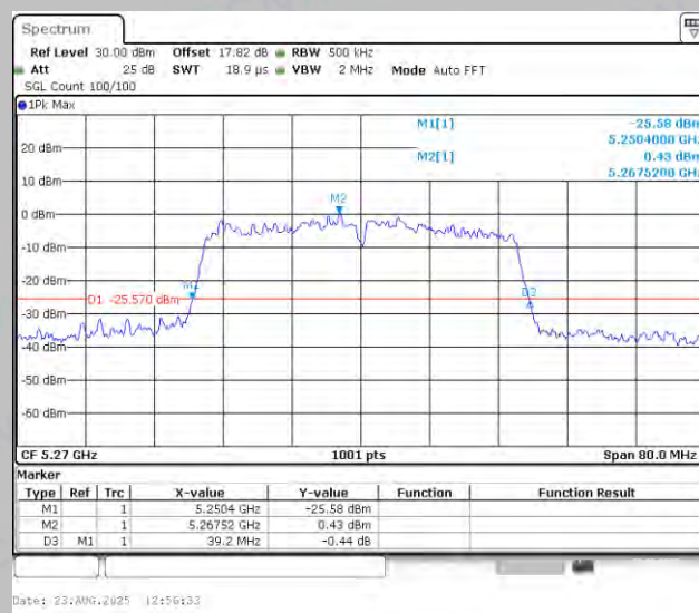
11N40MIMO-Ant2-5270
