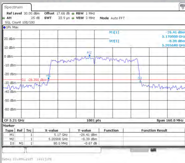
11AC80MIMO-Ant1-5210
