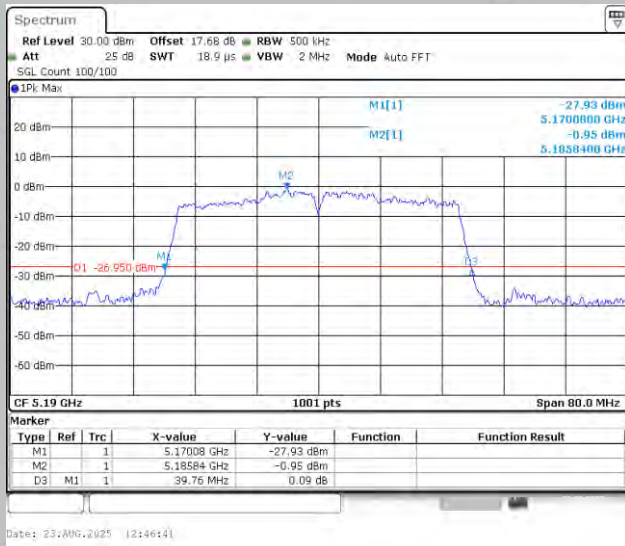
11N40MIMO-Ant1-5190
