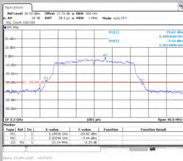
11N20MIMO-Ant2-5200
