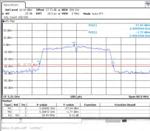
11N40MIMO-Ant1-5310
