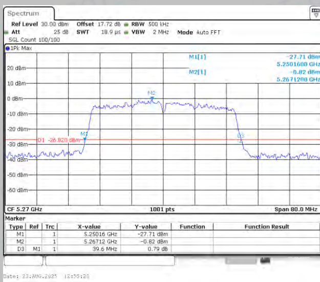
11N40MIMO-Ant1-5270
