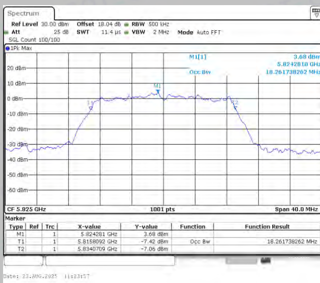
11N20MIMO-Ant1-5825
