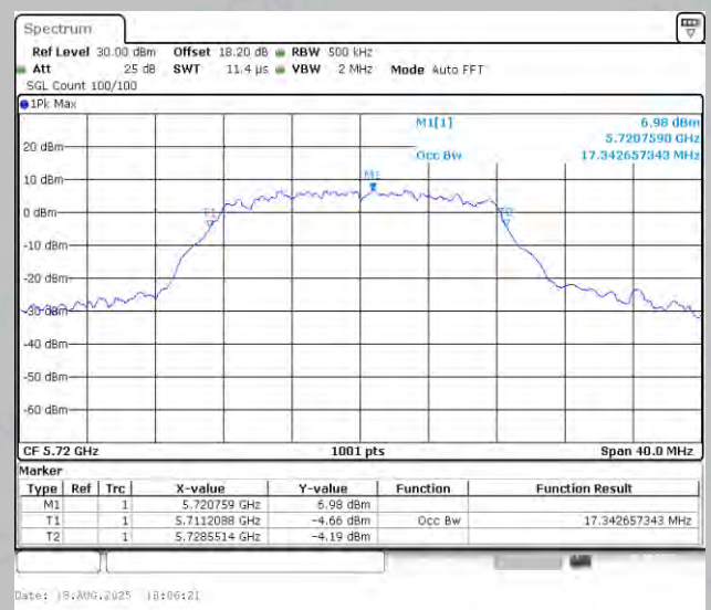
11A-Ant1-5720
