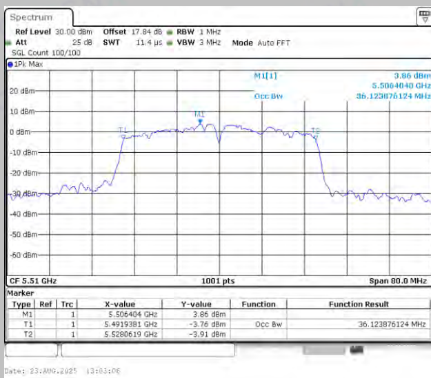
11N40MIMO-Ant1-5510
