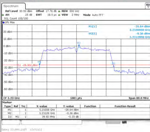
11N40MIMO-Ant1-5230
