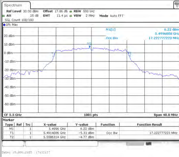
11A-Ant1-5500
