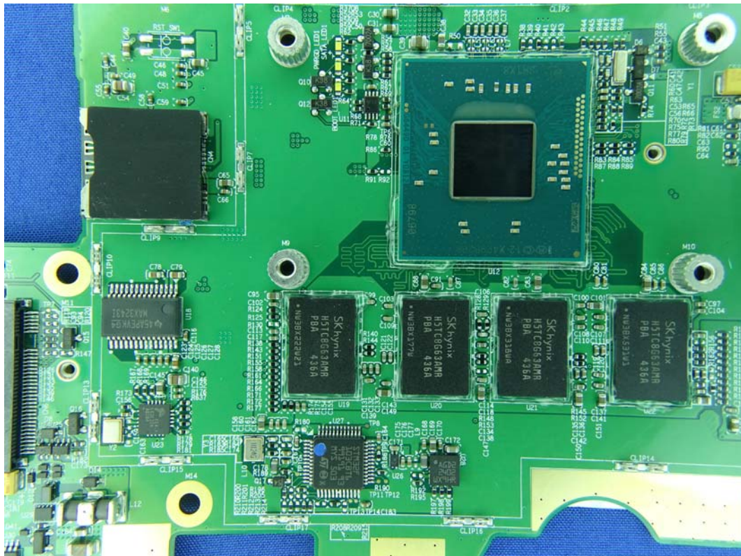
(69) EUT Photo
