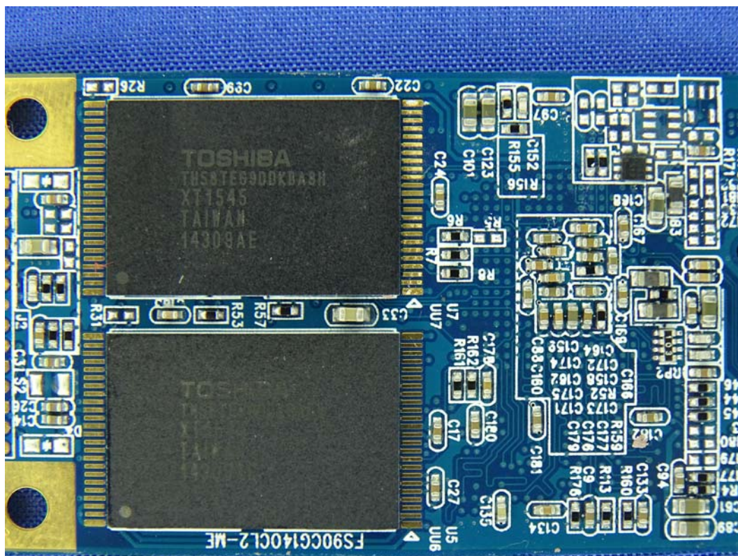
(67) EUT Photo
