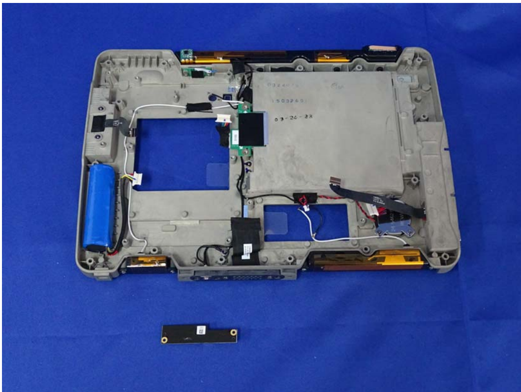
(72) EUT Photo
