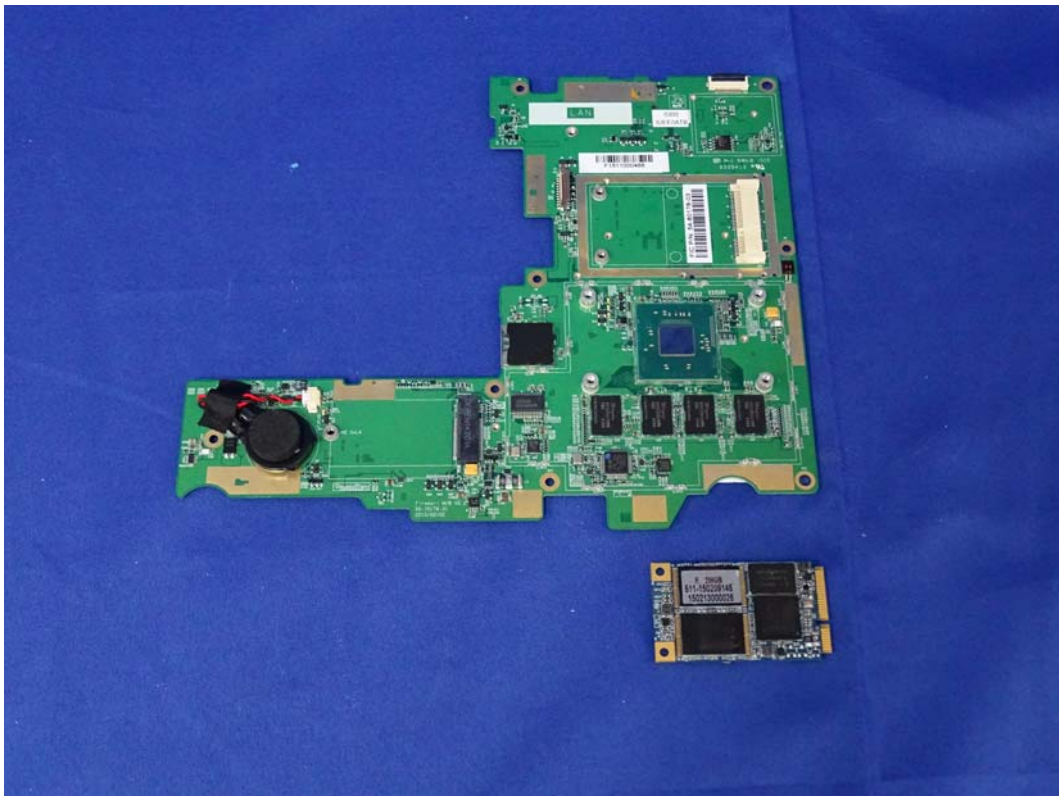
(63) EUT Photo
