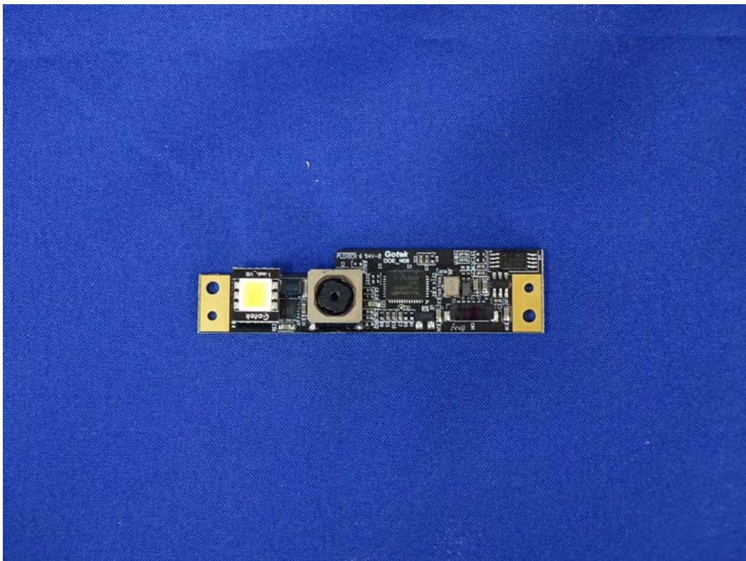
(74) EUT Photo
