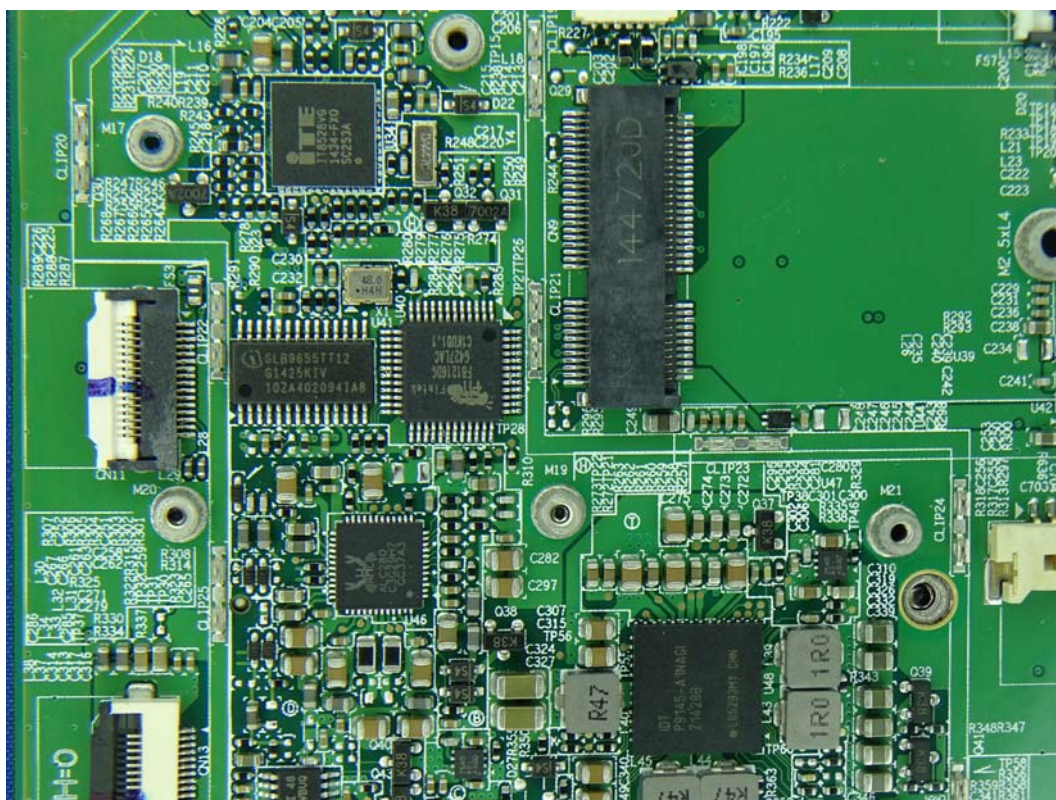
(54) EUT Photo
