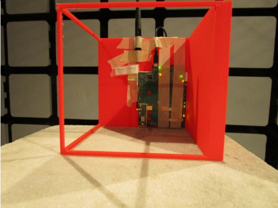
EUT Vertical
