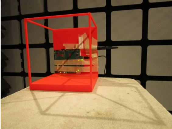
EUT Horizontal
