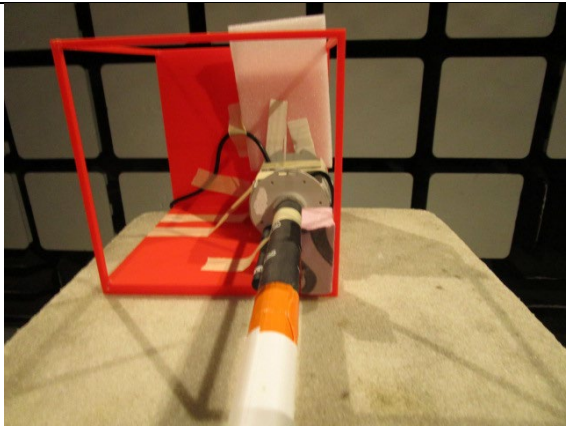
EUT Flat
