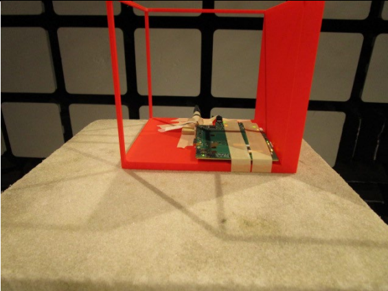
EUT Flat
