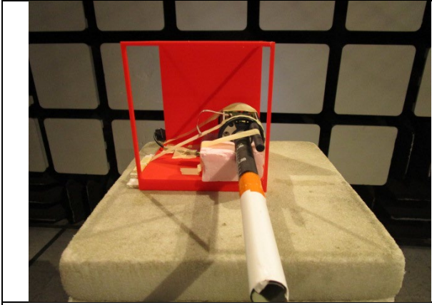
EUT Flat
