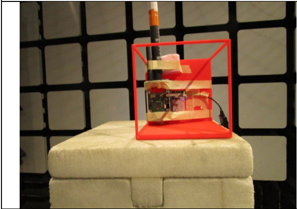
EUT Vertical
