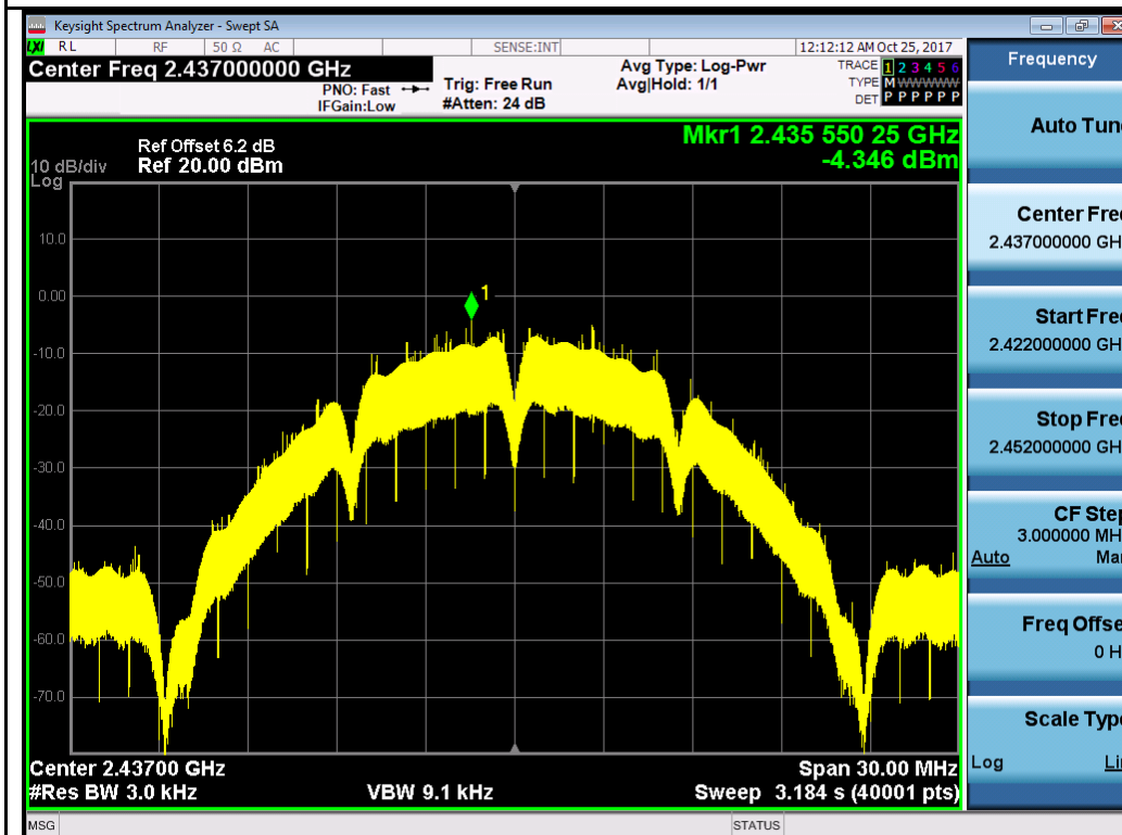
802.11b-2437MHz Chain 1
