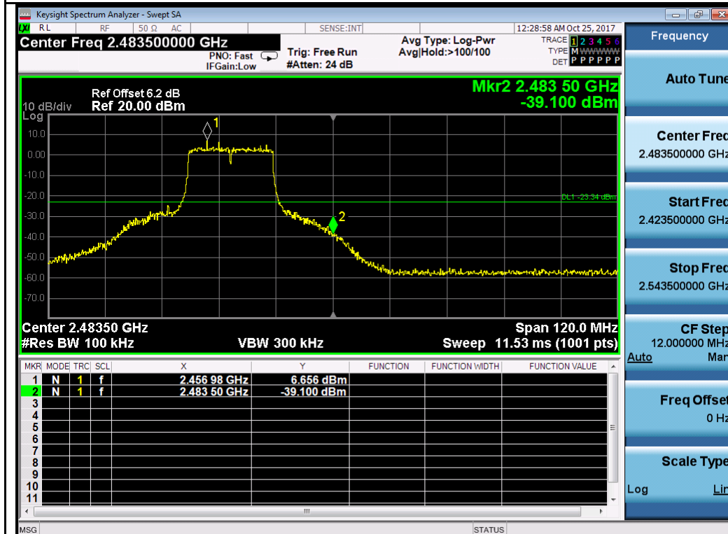
802.11n-HT20-2462MHz Chain 1
