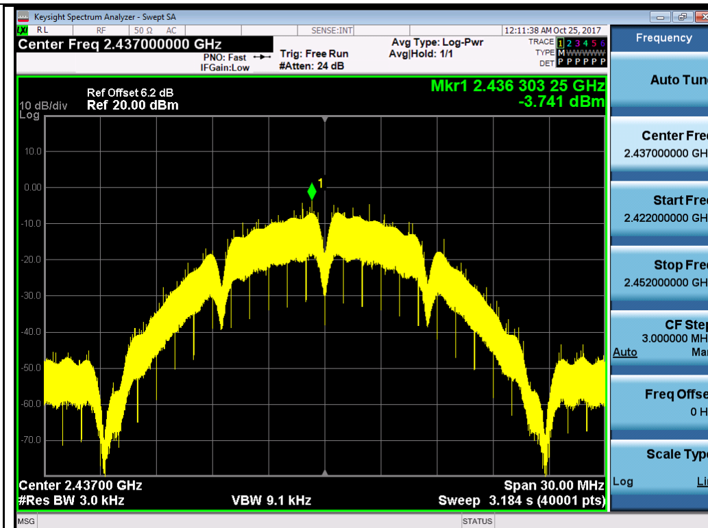
802.11b-2437MHz Chain 0
