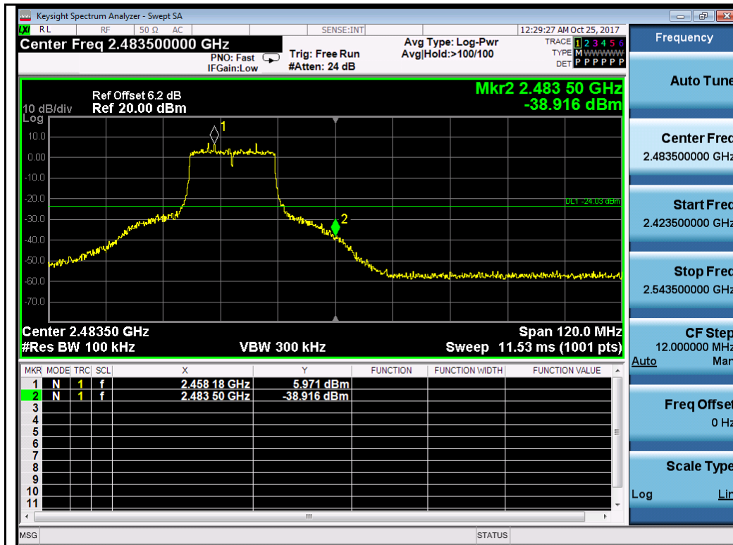
802.11n-HT20-2462MHz Chain 0
