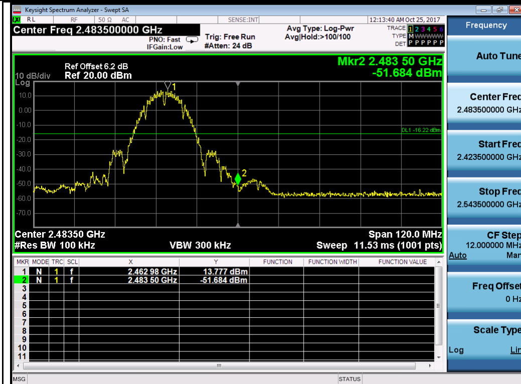
802.11b-2462MHz Chain 0
