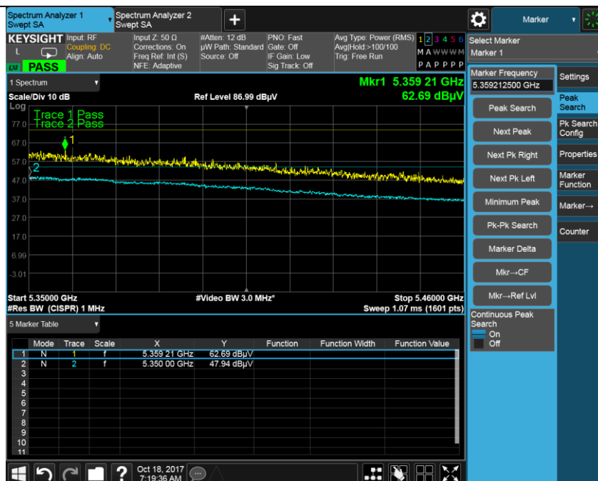
802.11ac 5290M(5350-5460MHz)
