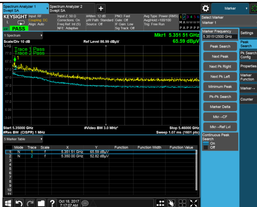
802.11n-HT40 5310M(5350-5460MHz)
