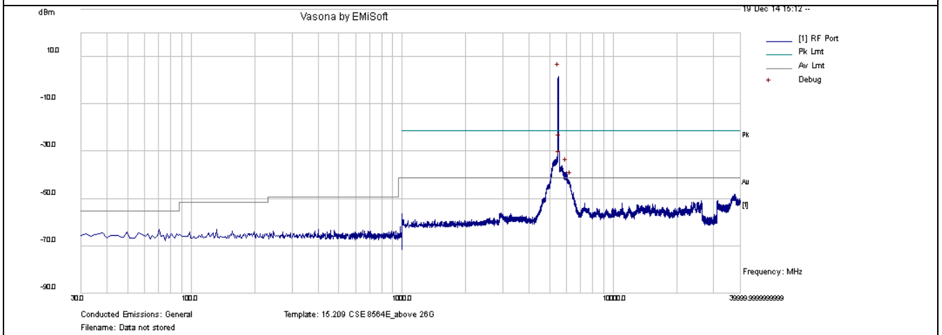
CSE-802.11a 5500MHz-chain1
