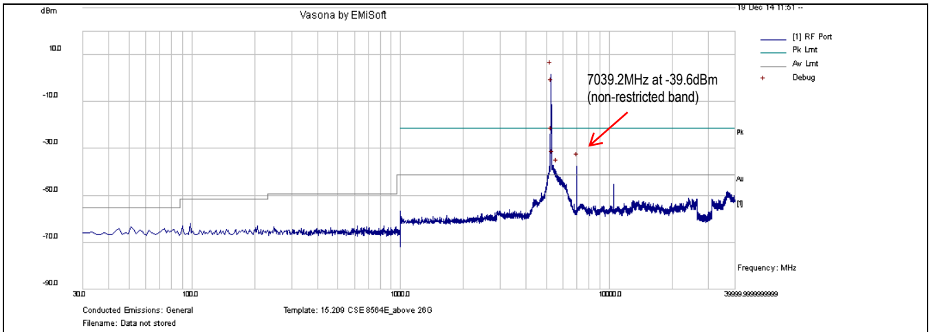
CSE-802.11n-20M 5280MHz-chain1
