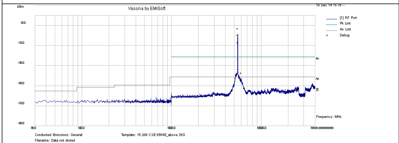
CSE-802.11n-20M 5500MHz-chain1
