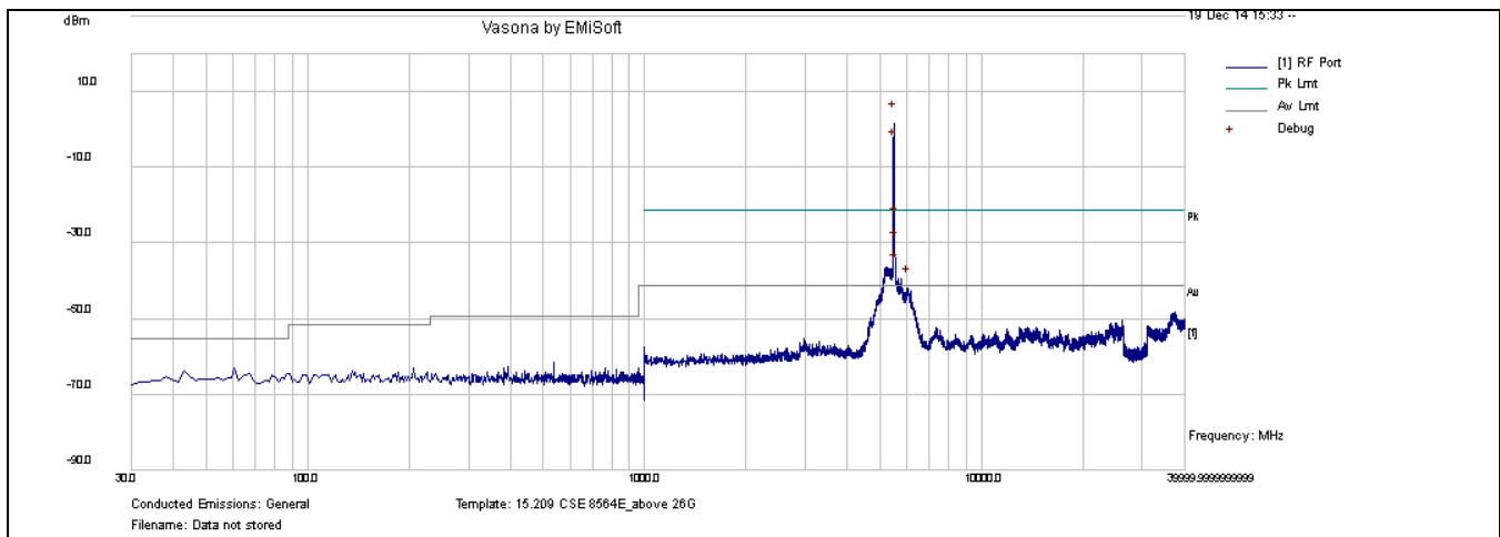
CSE-802.11n-20M 5500MHz-chain0
