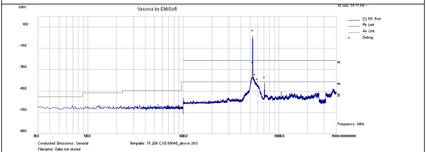
CSE-802.11n-20M 5320MHz-chain1
