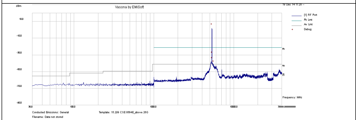
CSE-802.11a 5320MHz-chain0
