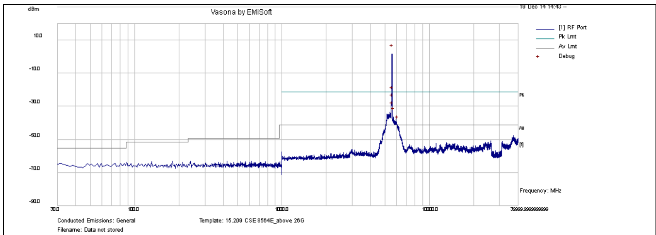
CSE-802.11a 5580MHz-chain1
