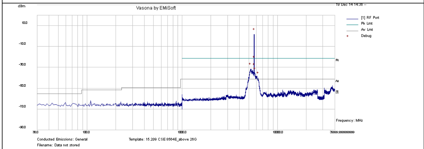
CSE-802.11a 5700MHz-chain0
