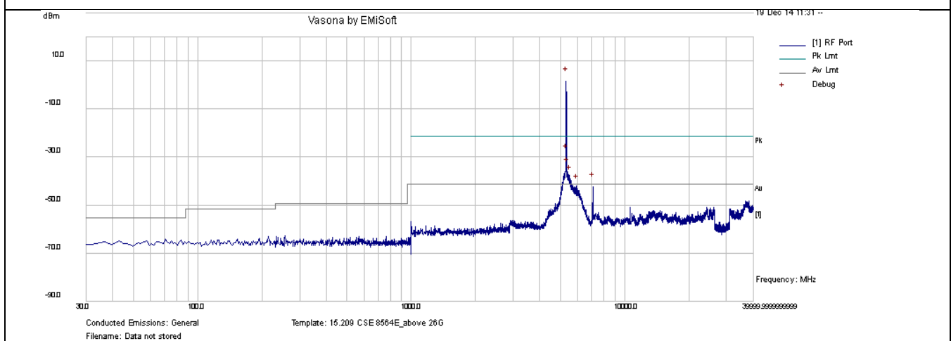
CSE-802.11a 5320MHz-chain1
