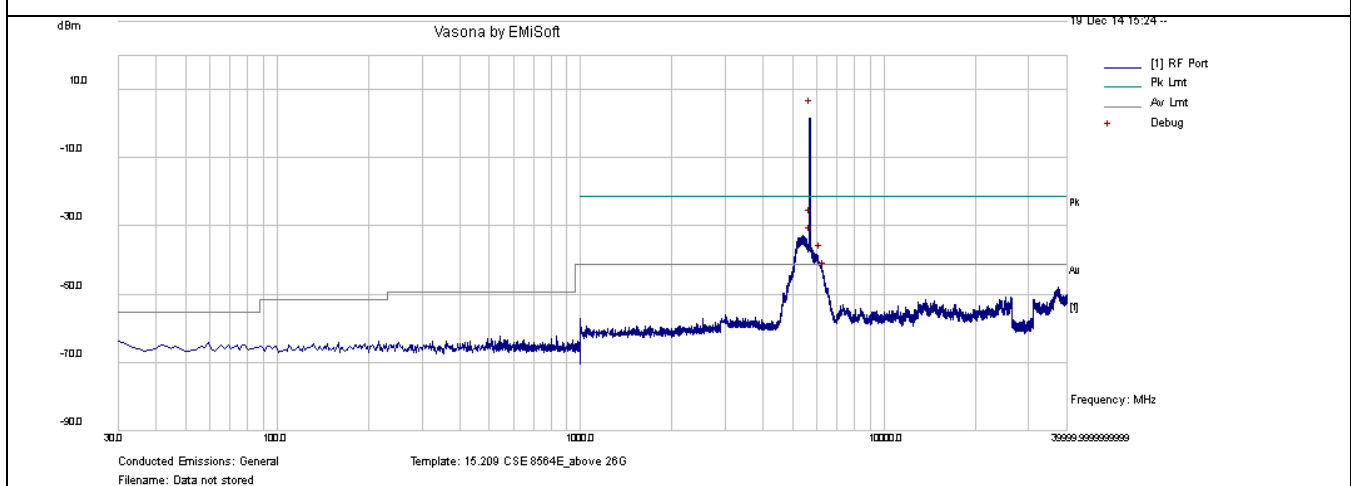
CSE-802.11n-20M 5700MHz-chain1
