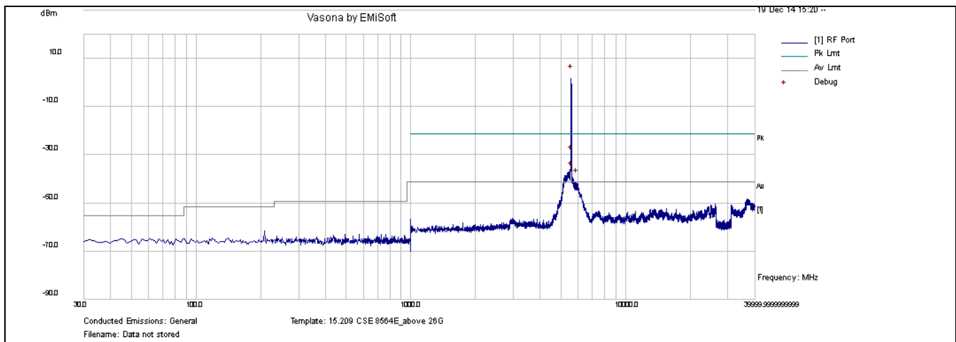
CSE-802.11n-20M 5580MHz-chain1
