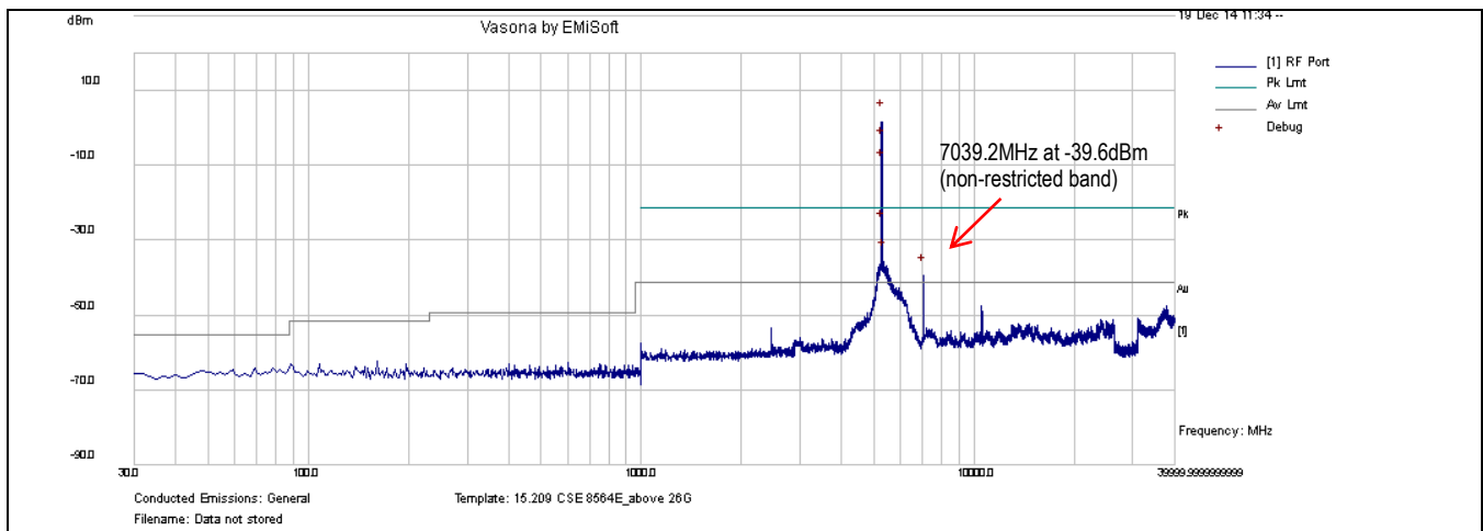
CSE-802.11a 5280MHz-chain1
