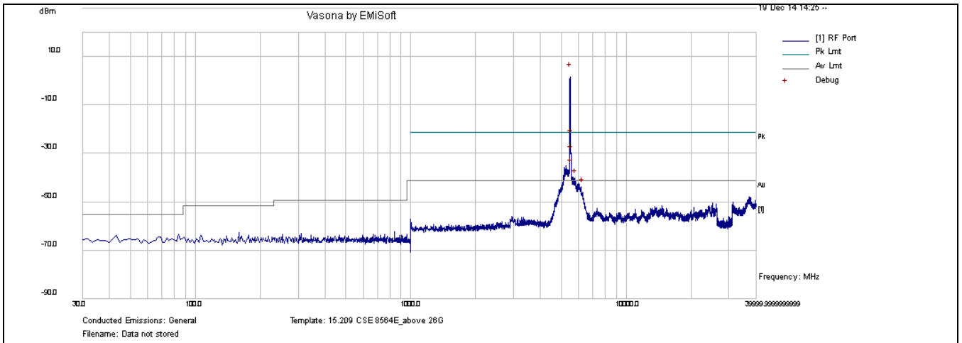
CSE-802.11a 5500MHz-chain0
