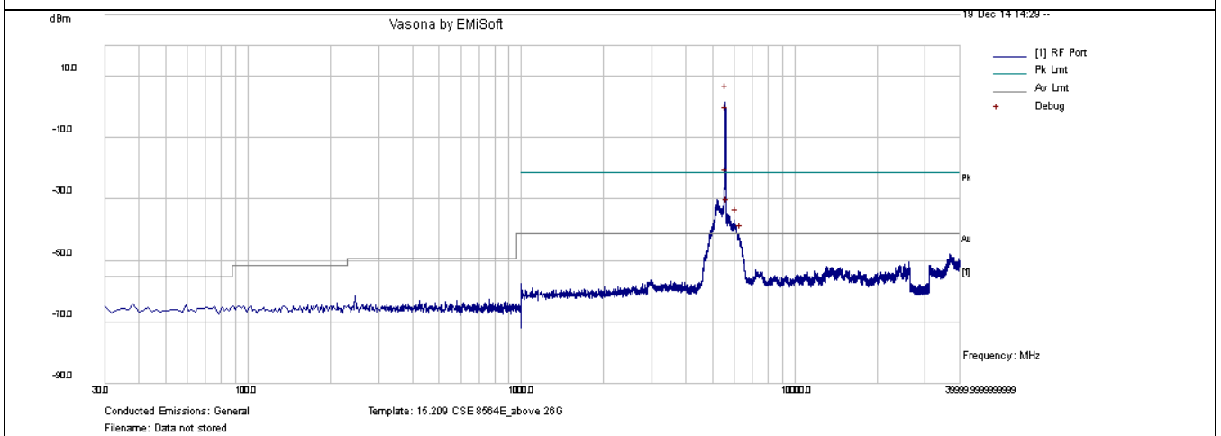
CSE-802.11a 5580MHz-chain0
