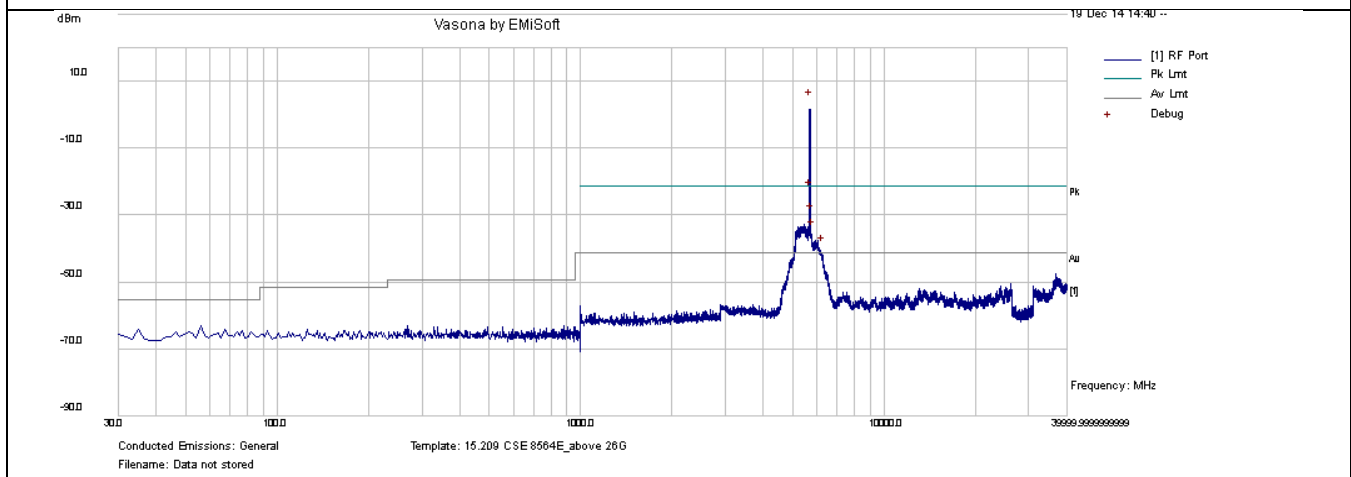
CSE-802.11a 5700MHz-chain1
