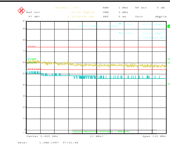
802.11ac-VHT80 5290M(5350-5460MHz)
