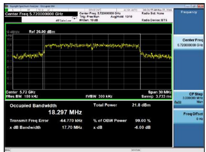
6dB BW -802.11n-20M 5720MHz
