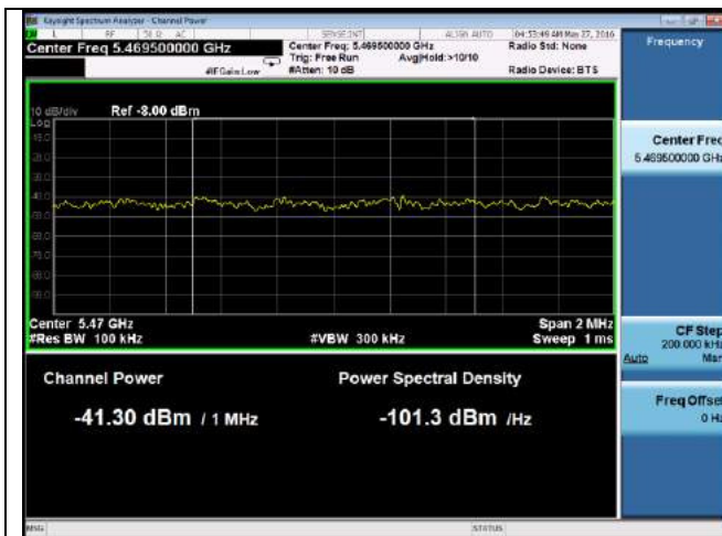
Band Edge -802.11a-5500M-chain0
