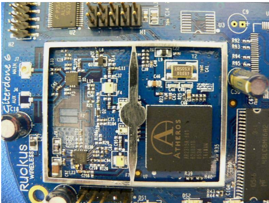
MM22X1: EUT – TX Close Up
