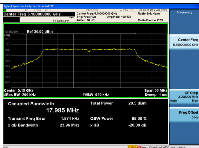
26dB BW - 802.11n-HT20 5180MHz
