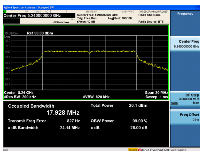
26dB BW - 802.11n-HT20 5240MHz
