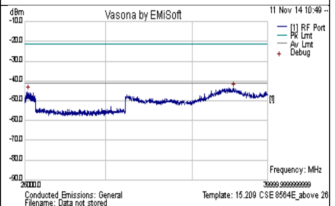
CSE-802.11n-20M-5320MHz-above 26GHz-chain1
