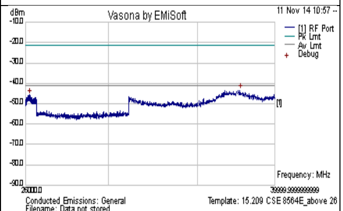
CSE-802.11n-20M-5700MHz-above 26GHz-chain1
