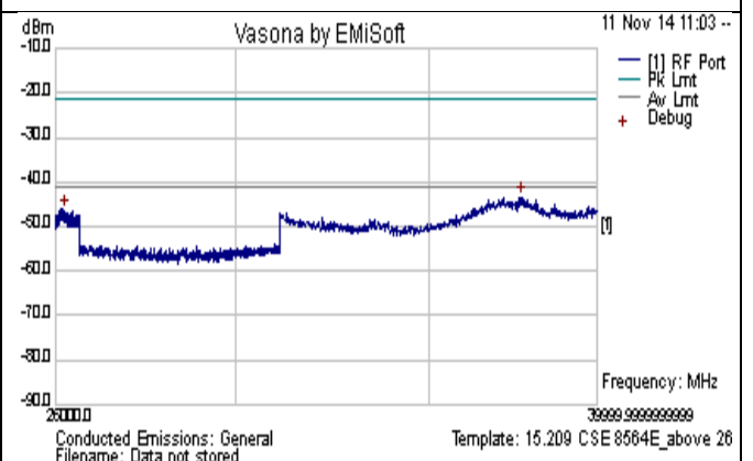
CSE-802.11ac-80M-5610MHz-above 26GHz-chain1
