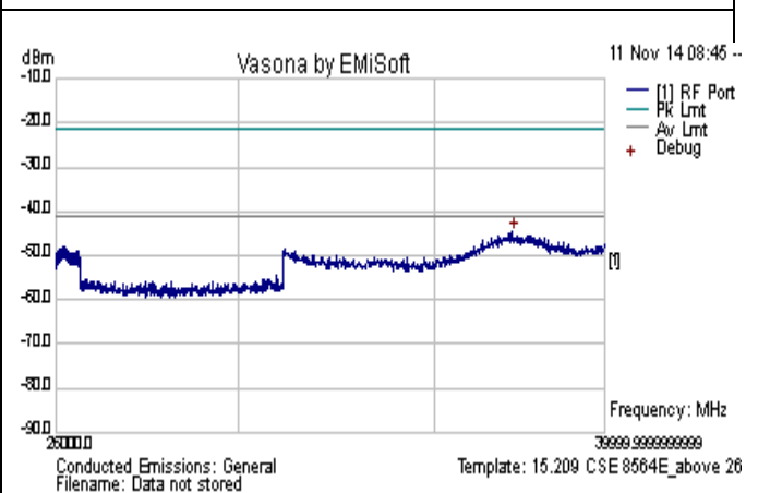
CSE-802.11n-20M-5260MHz-above 26GHz-chain1
