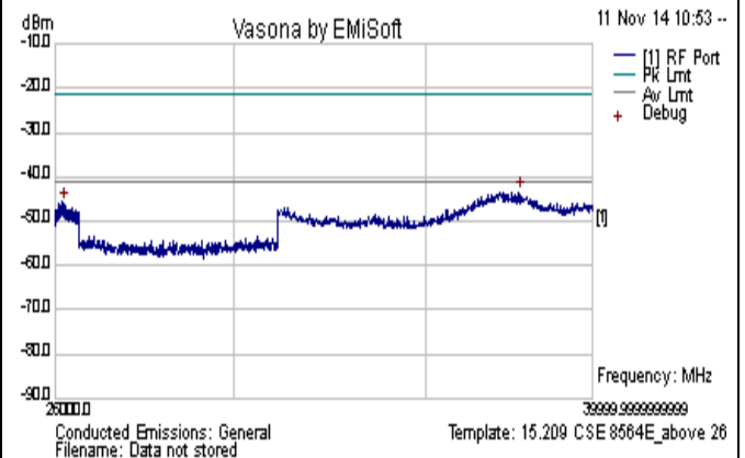
CSE-802.11n-20M-5500MHz-above 26GHz-chain2
