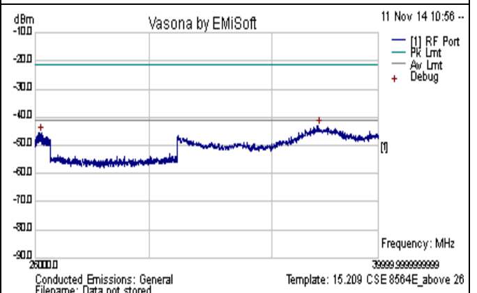
CSE-802.11n-20M-5580MHz-above 26GHz-chain2
