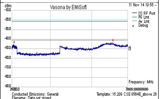
CSE-802.11n-20M-5580MHz-above 26GHz-chain1
