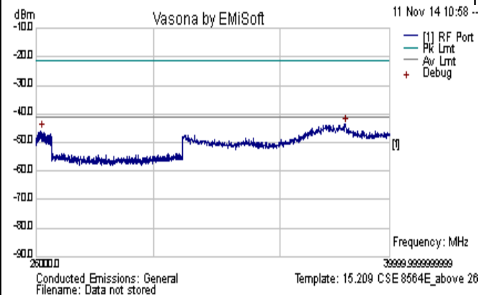
CSE-802.11n-20M-5700MHz-above 26GHz-chain2
