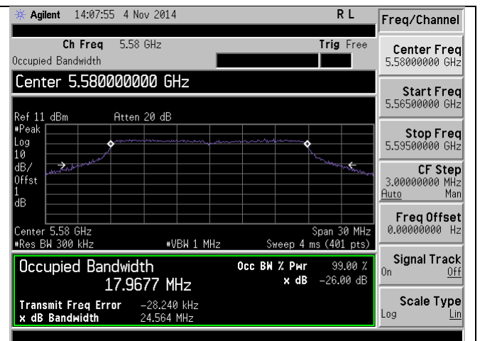
26dB BW -802.11n-20M 5580MHz
