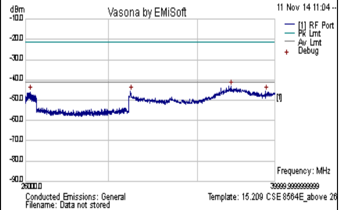
CSE-802.11ac-80M-5610MHz-above 26GHz-chain2
