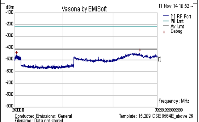
CSE-802.11n-20M-5500MHz-above 26GHz-chain1
