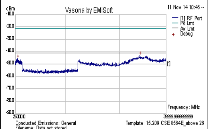
CSE-802.11n-20M-5300MHz-above 26GHz-chain2
