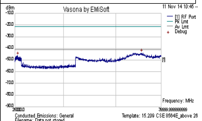
CSE-802.11n-20M-5300MHz-above 26GHz-chain1
