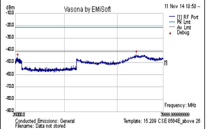
CSE-802.11n-20M-5320MHz-above 26GHz-chain2
