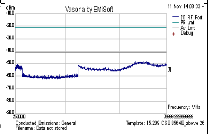
CSE-802.11a 5320MHz-above 26GHz-chain1
