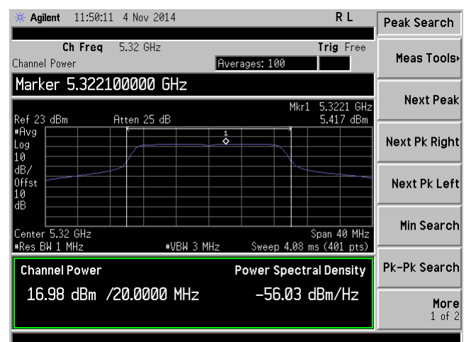
PSD-802.11n-20M-5320M-chain2
