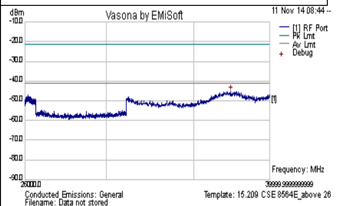
CSE-802.11n-20M-5260MHz-above 26GHz-chain1
