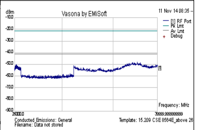
CSE-802.11a 5320MHz-above 26GHz-chain2
