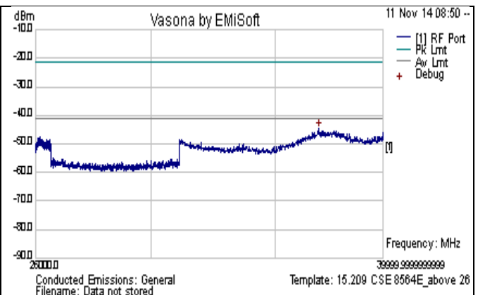
CSE-802.11n-20M-5700MHz-above 26GHz-chain0
