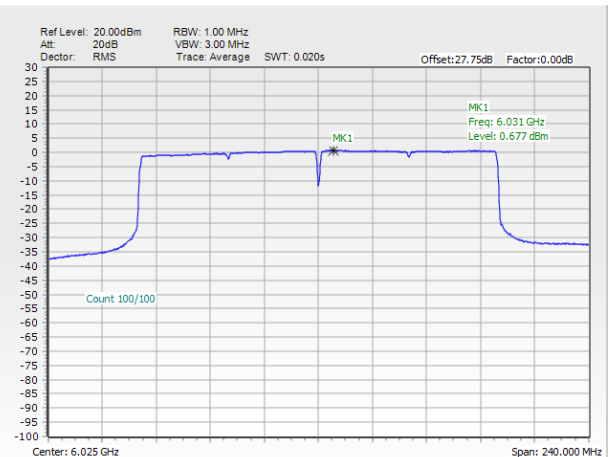
MIMO Ant. 2
