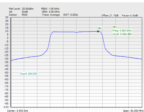
MIMO Ant. 2
