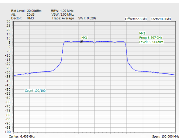
MIMO Ant. 2
