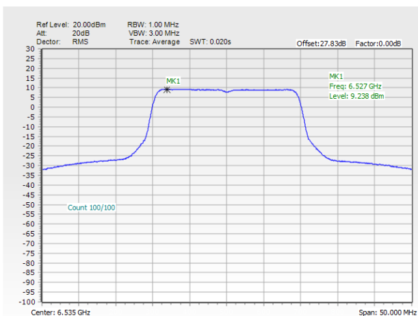
MIMO Ant. 4
