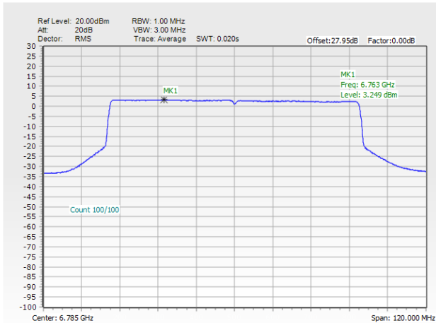
MIMO Ant. 4
