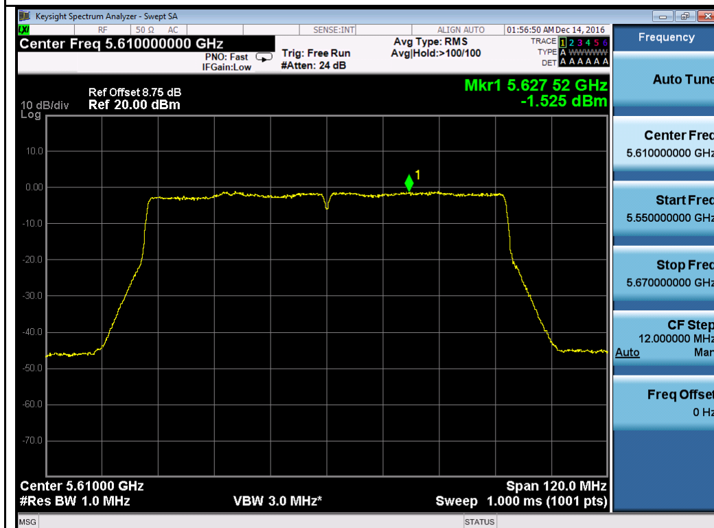
802.11ac-VHT80 5610M
