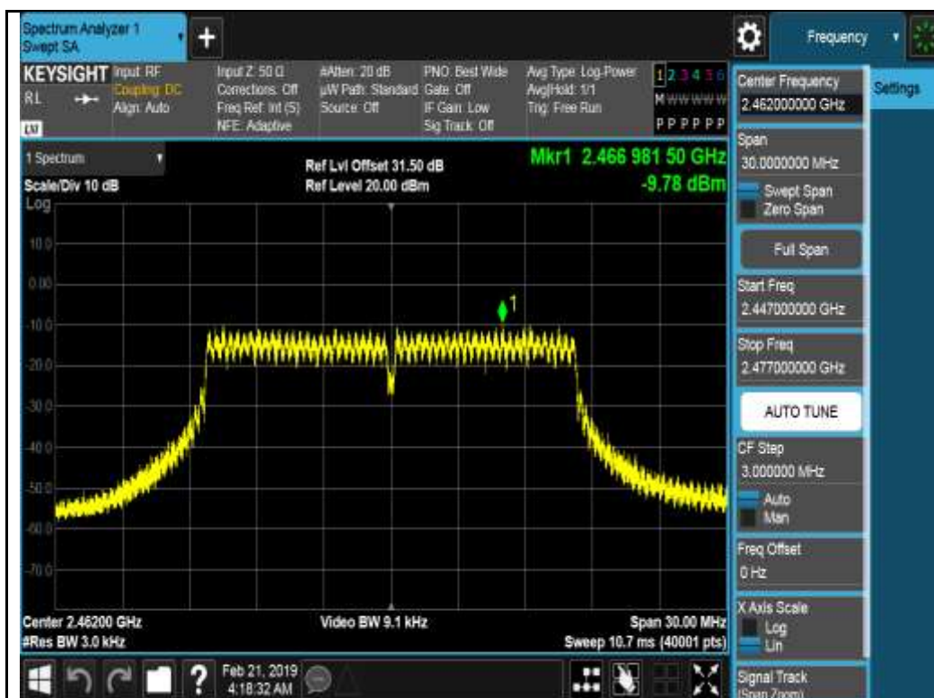
802.11g-2462MHz Chain 2
