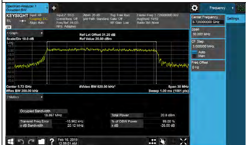
802.11ax-HT20 5720MHz
