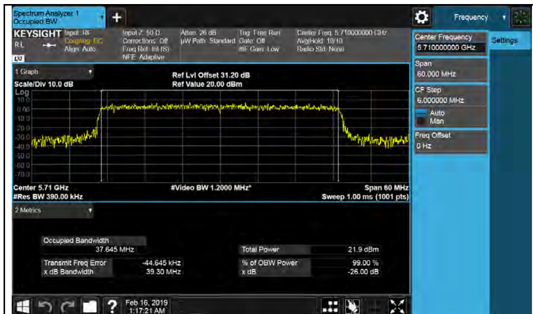
802.11ax-HT40 5710MHz
