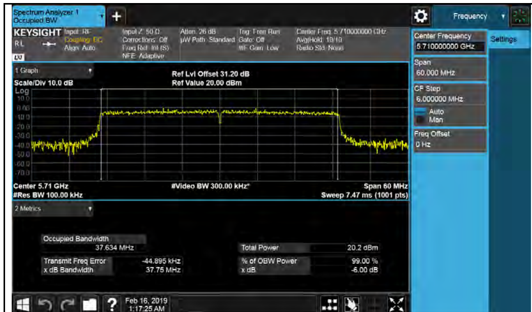
802.11ax-HT40 5710MHz
