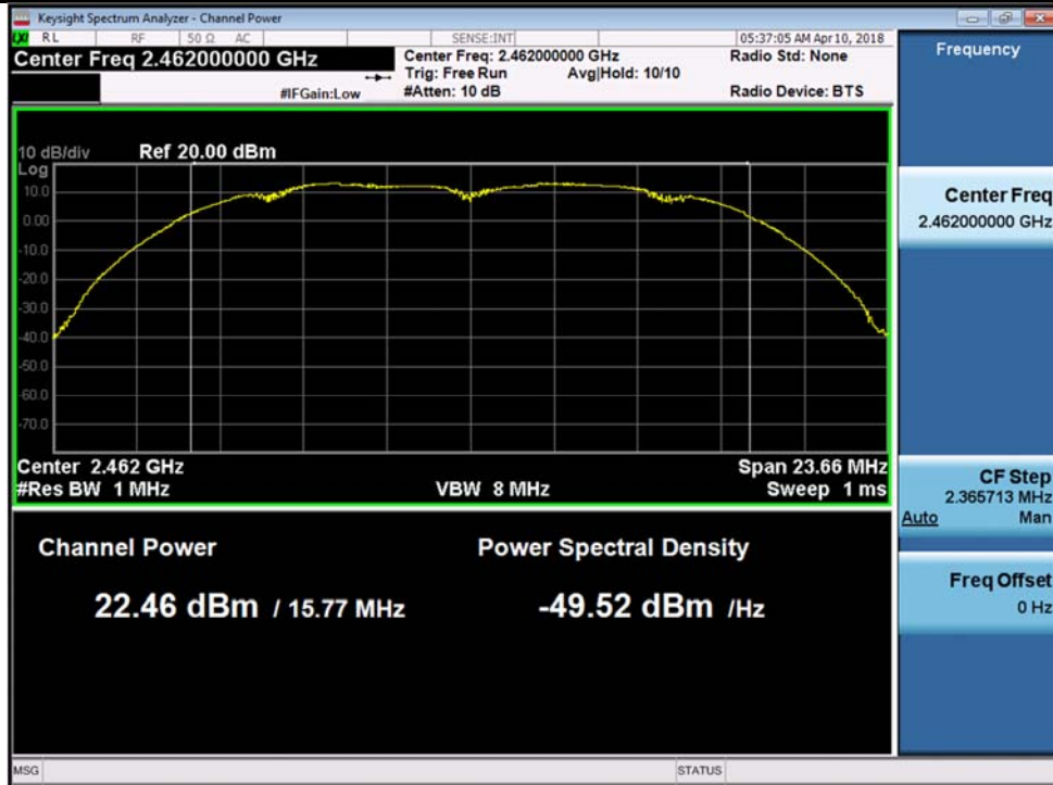
802.11b-2462MHz Chain 2
