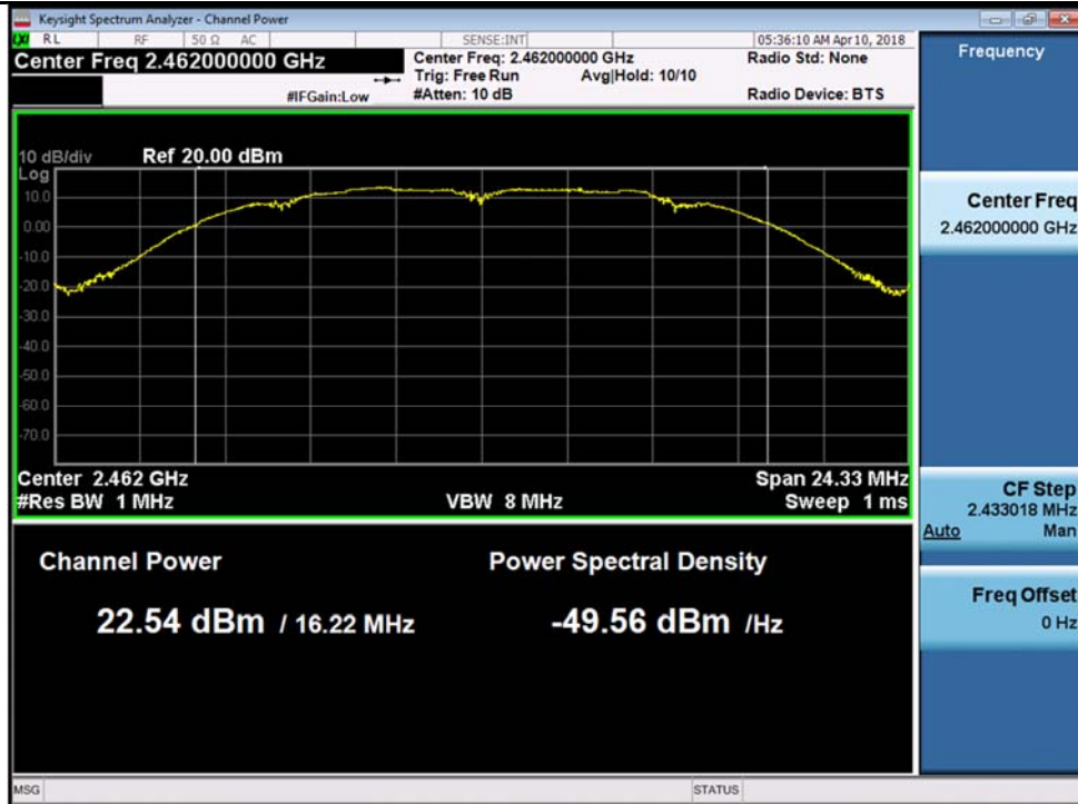
802.11b-2462MHz Chain 1
