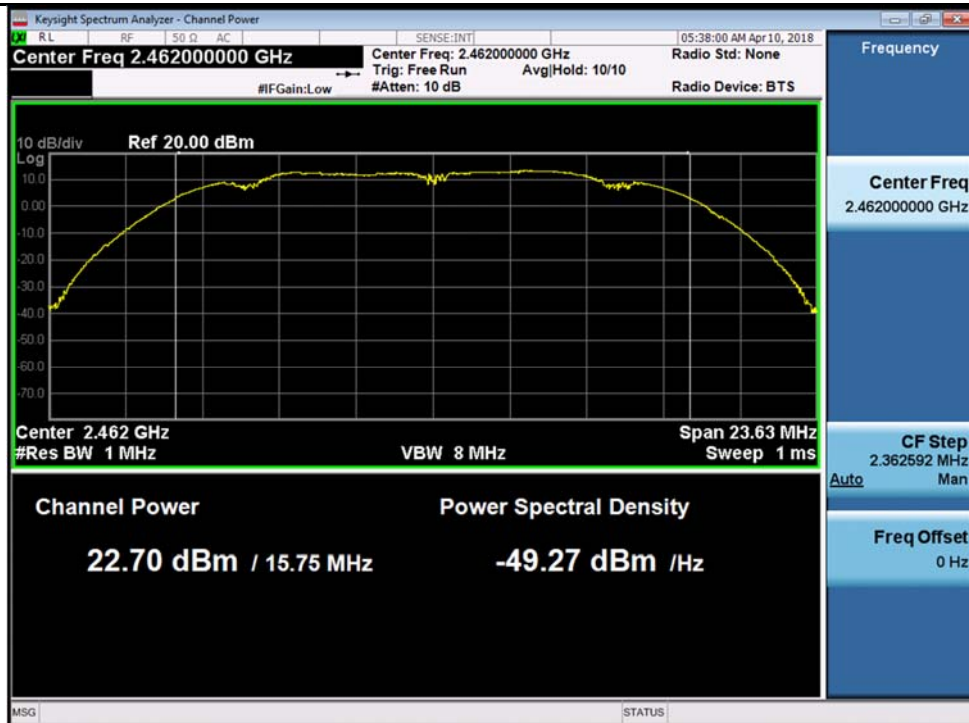
802.11b-2462MHz Chain 3
