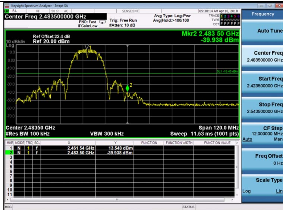
802.11b-2462MHz Chain 3
