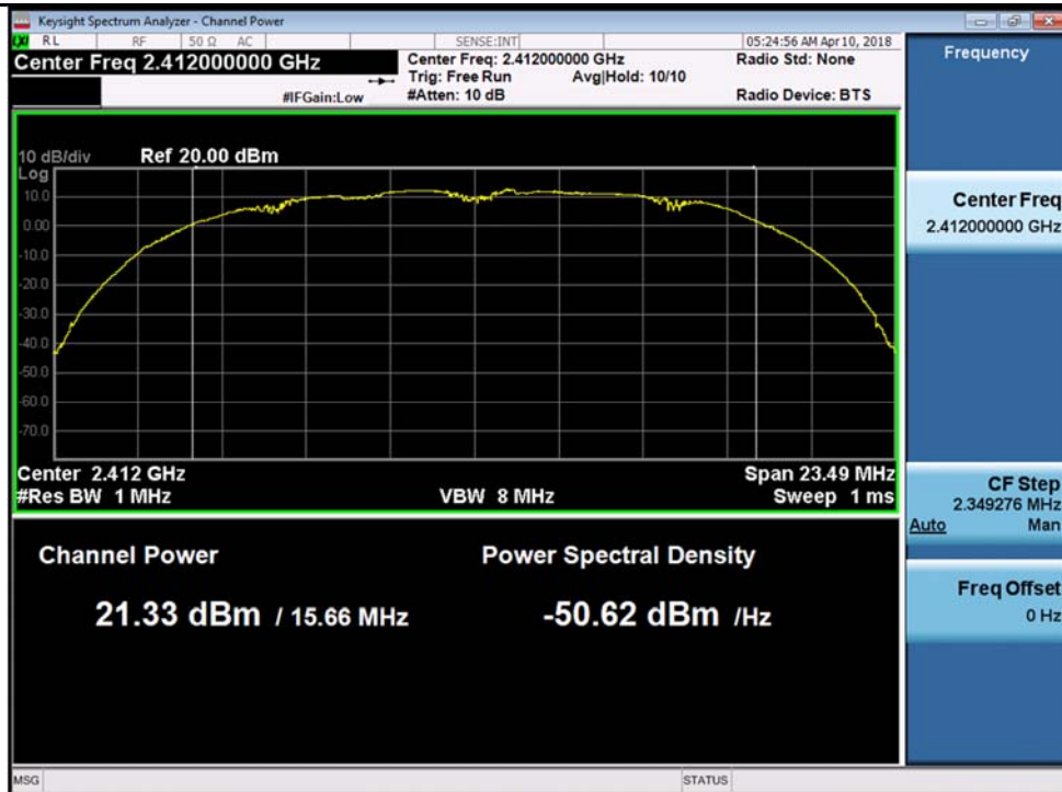
802.11b-2412MHz Chain 3
