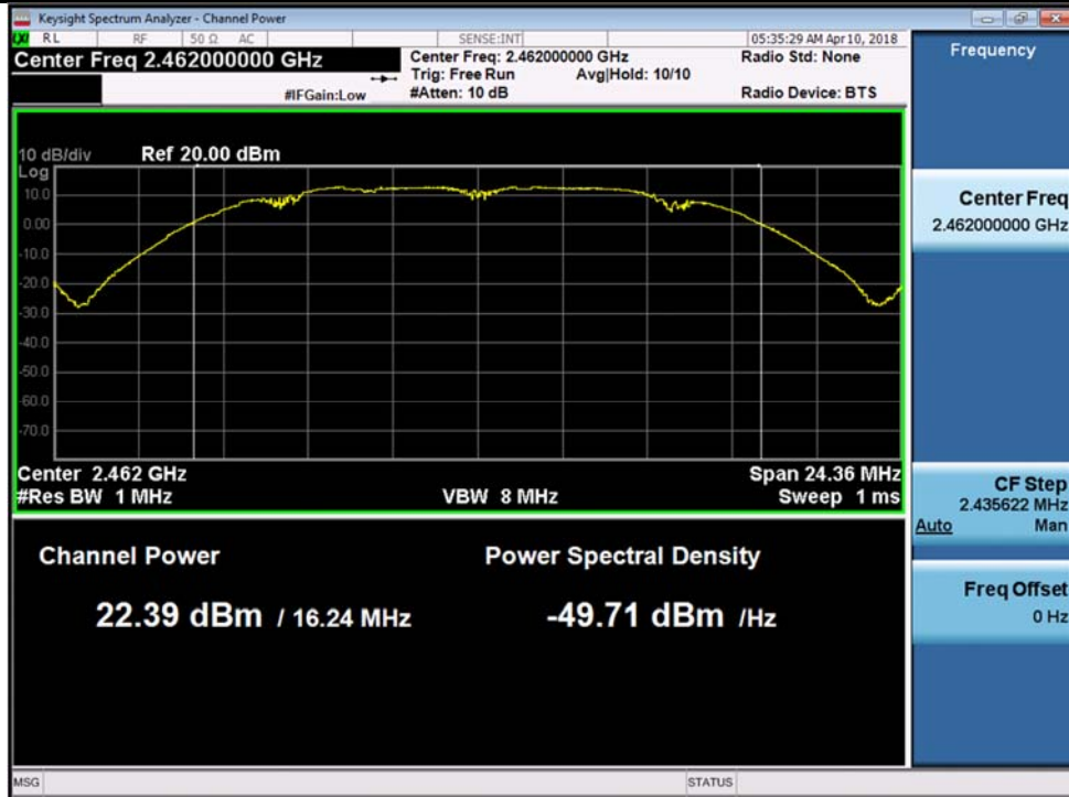
802.11b-2462MHz Chain 0
