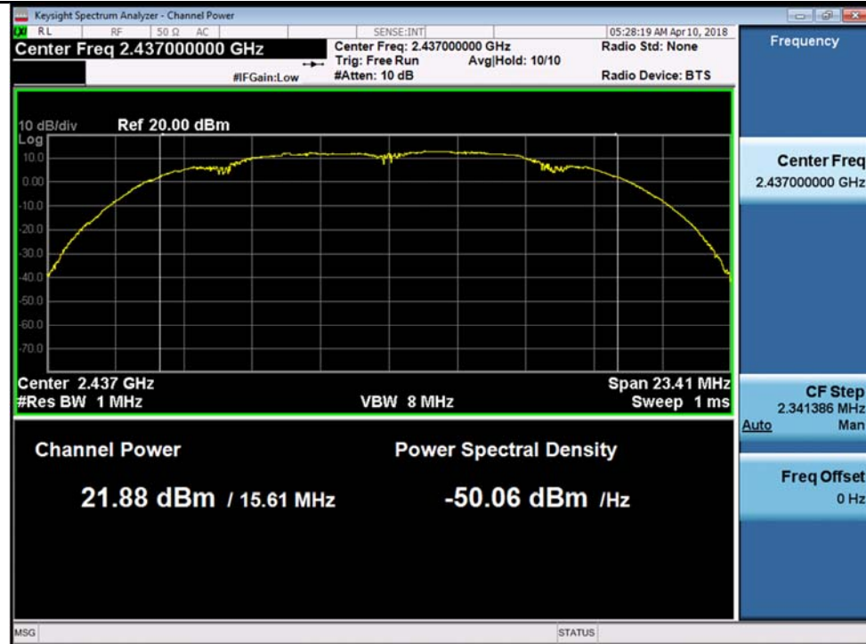
802.11b-2437MHz Chain 3
