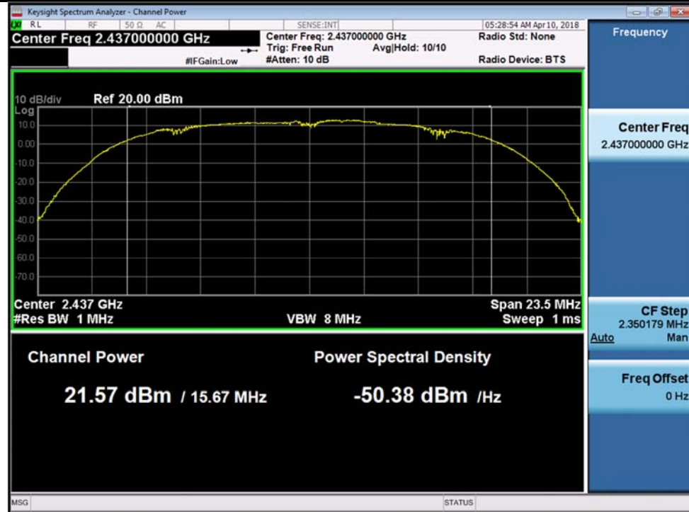
802.11b-2437MHz Chain 2
