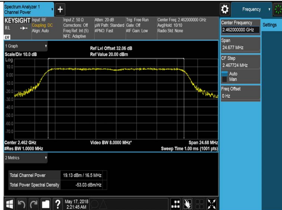
802.11g-2462MHz Chain 3
