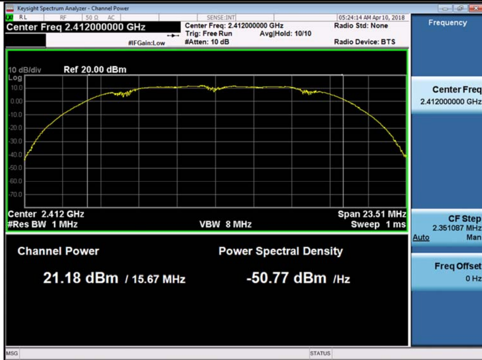
802.11b-2412MHz Chain 2
