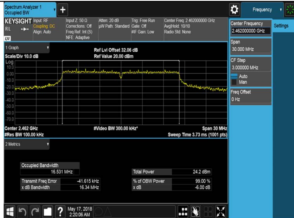
802.11g-2462MHz
