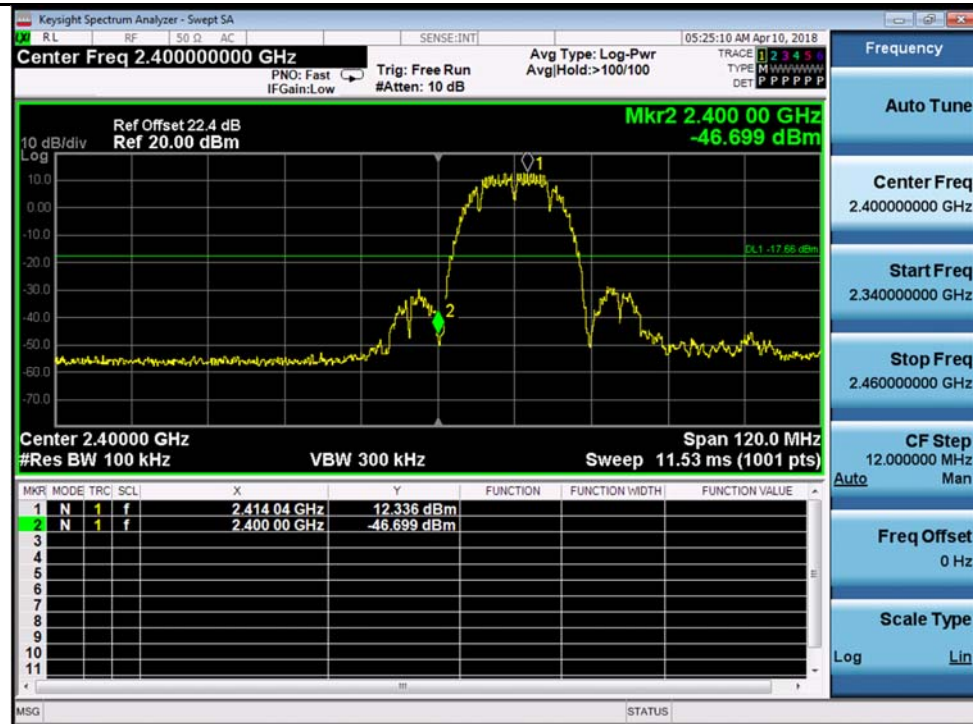
802.11b-2412MHz Chain 3
