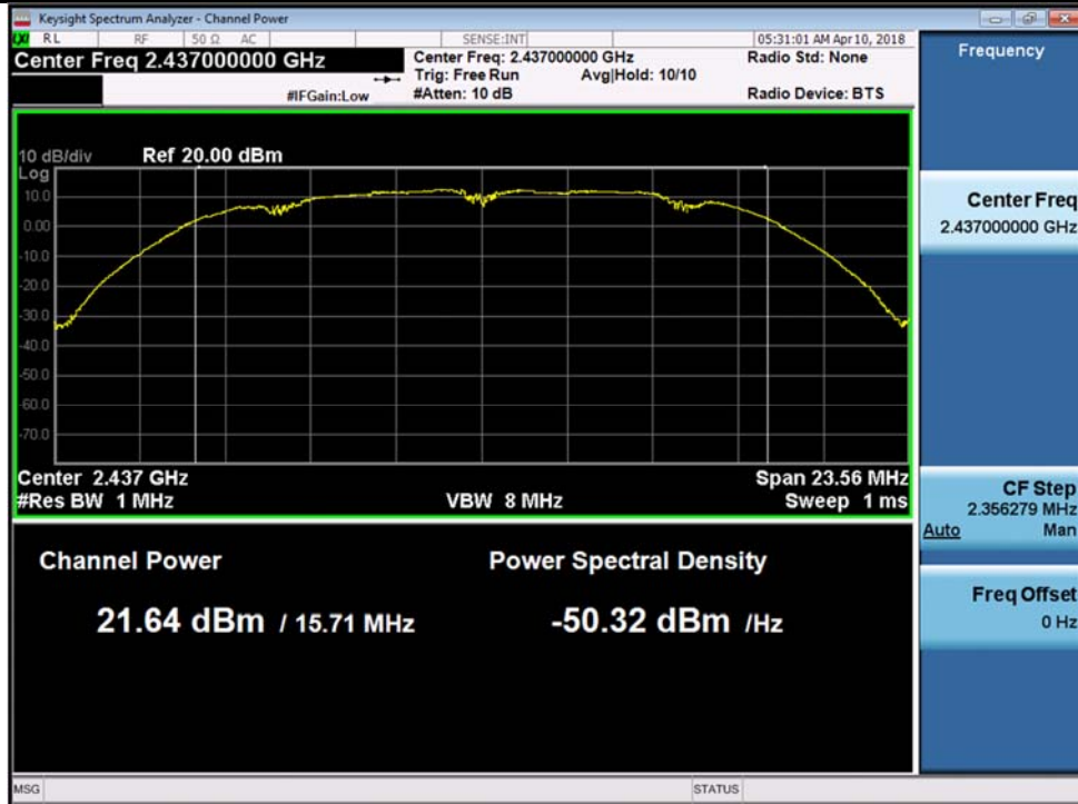
802.11b-2437MHz Chain 0
