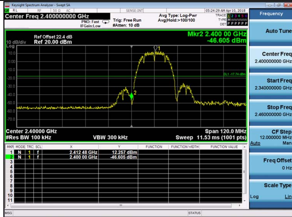
802.11b-2412MHz Chain 2
