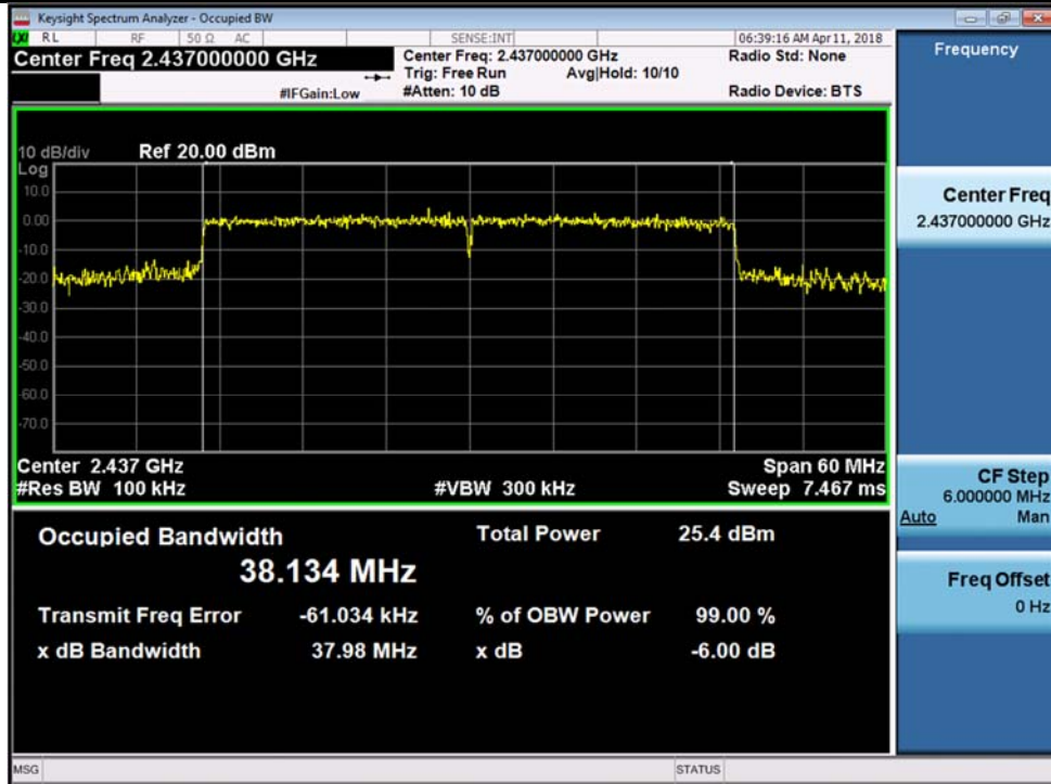
802.11ax40-2437MHz
