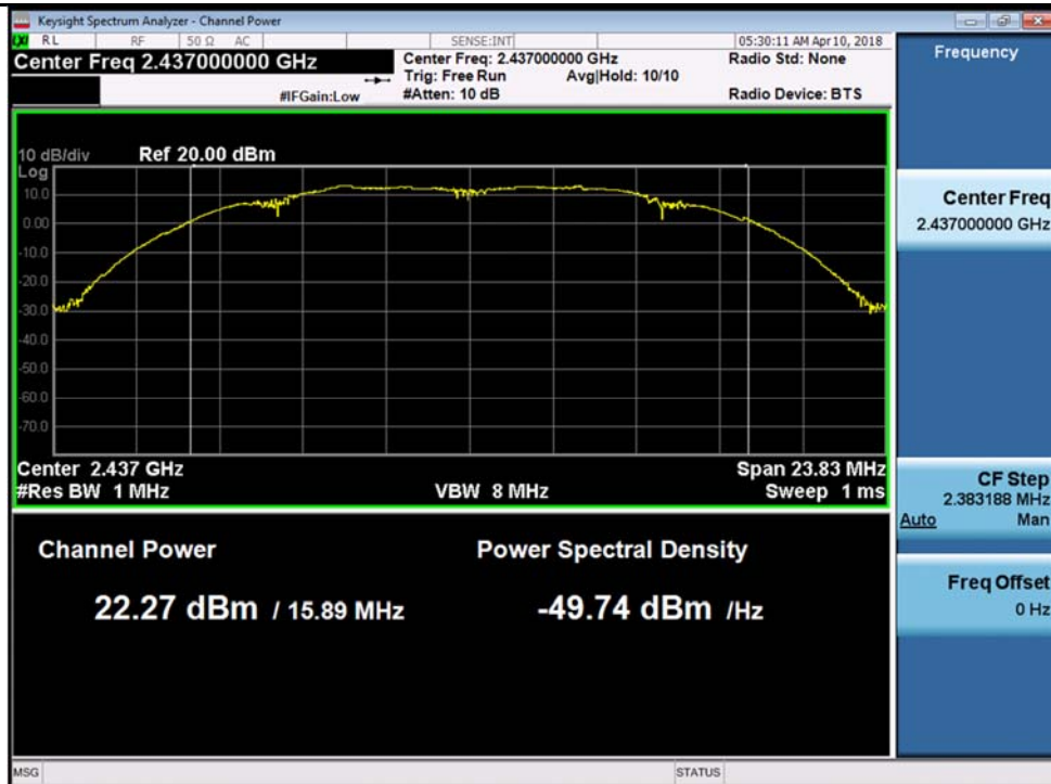
802.11b-2437MHz Chain 1
