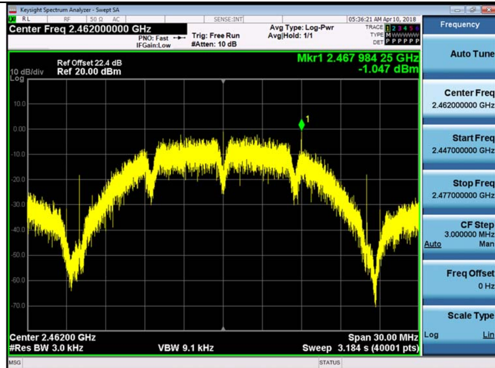
802.11b-2462MHz Chain 1
