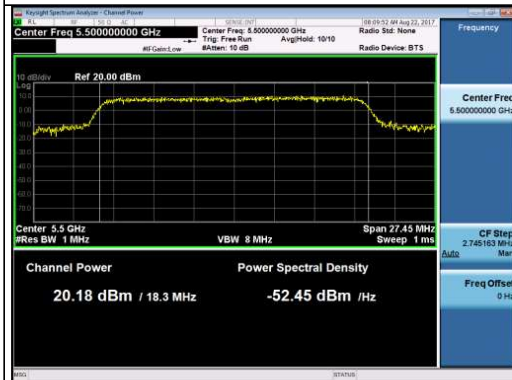
802.11n-HT20 5500M
