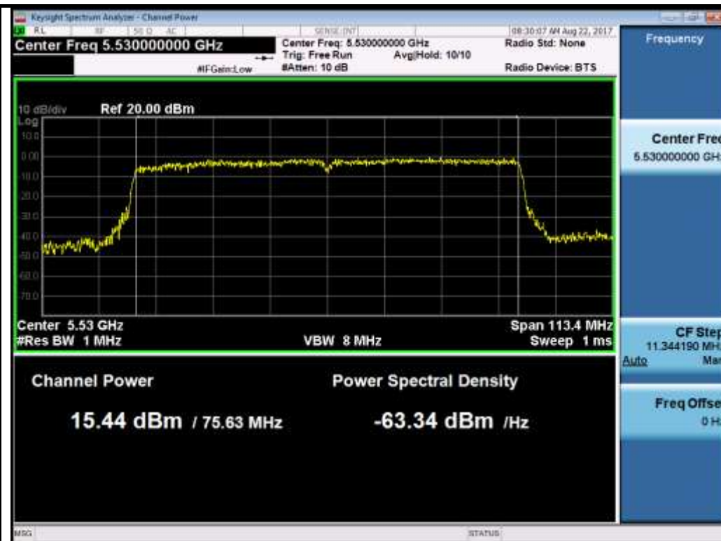
802.11ac-VHT80 5530M
