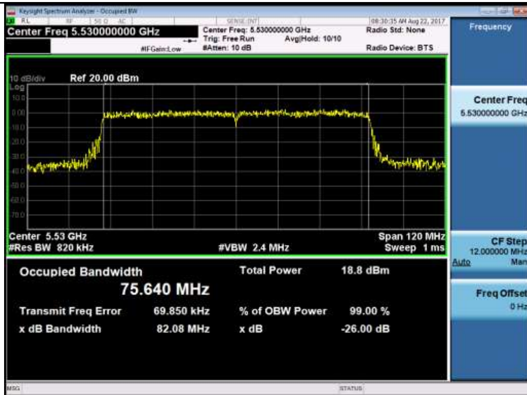
802.11ac-VHT80-5530MHz
