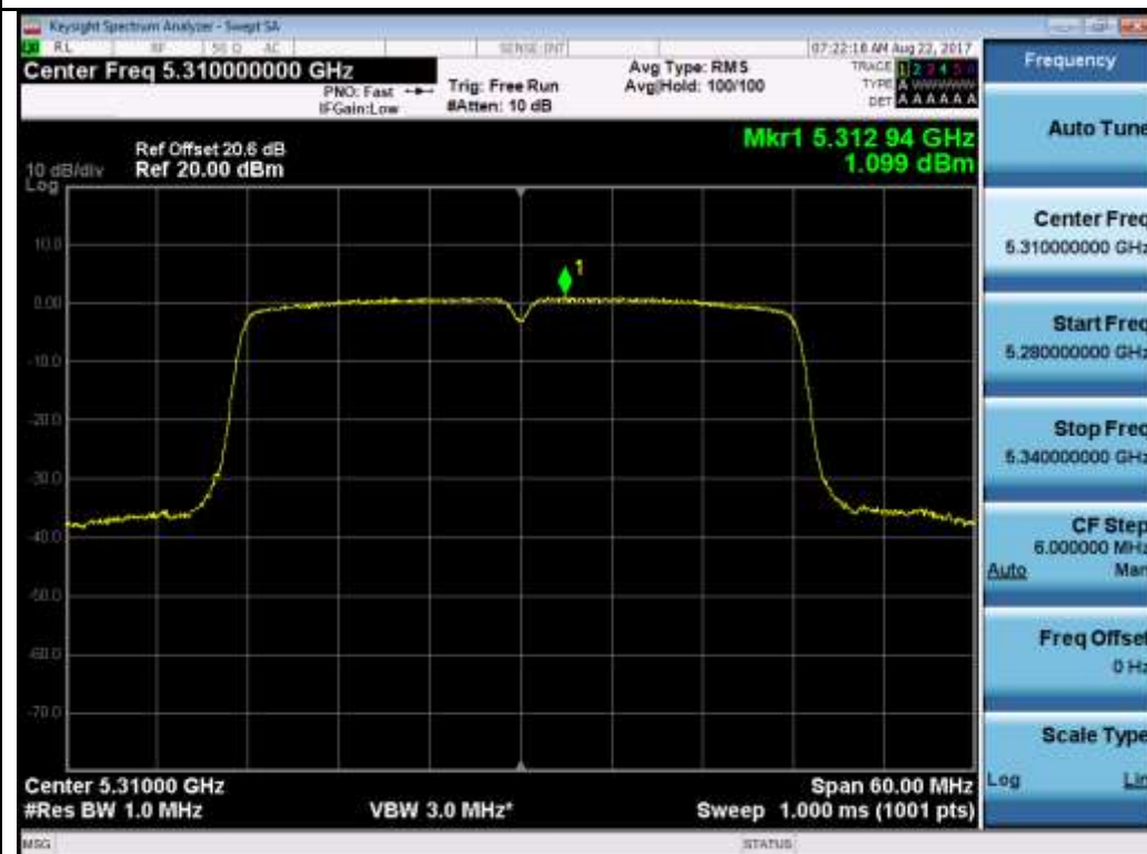
802.11n-HT40 5310M
