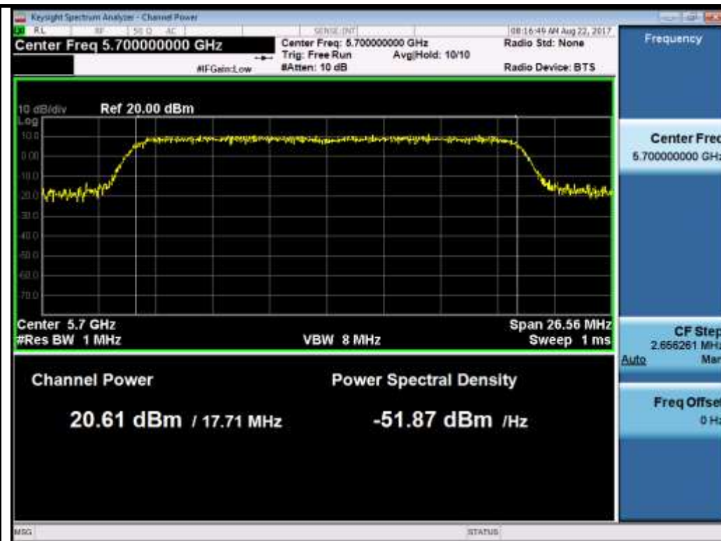
802.11n-HT20 5700M
