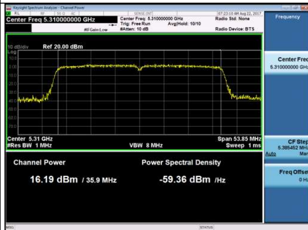
802.11n-HT40 5310M
