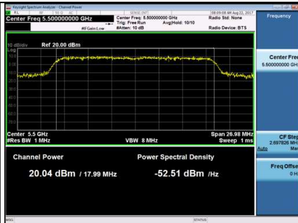
802.11n-HT20 5500M
