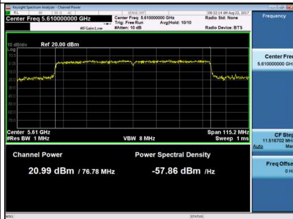
802.11ac-VHT80 5610M
