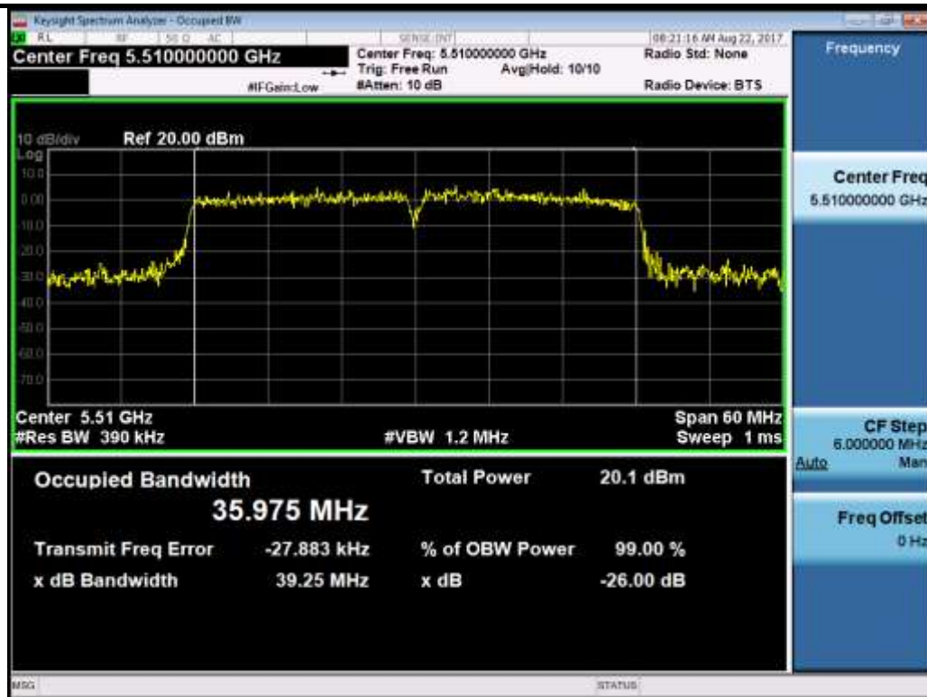
802.11n-HT40-5510MHz
