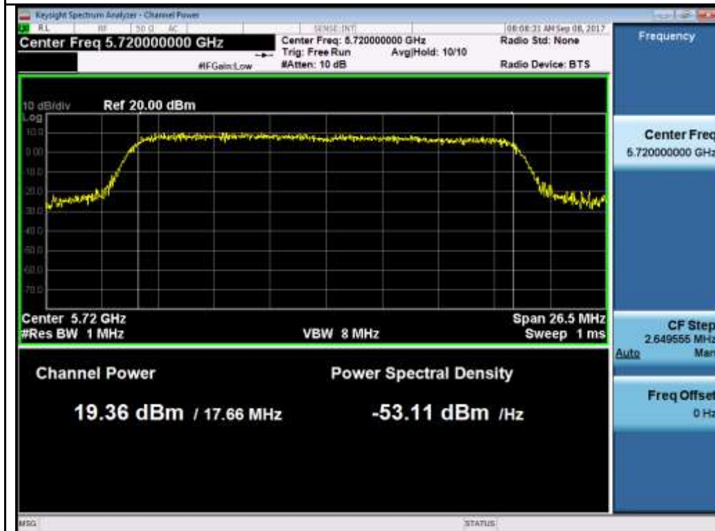
802.11n-HT20 5720M
