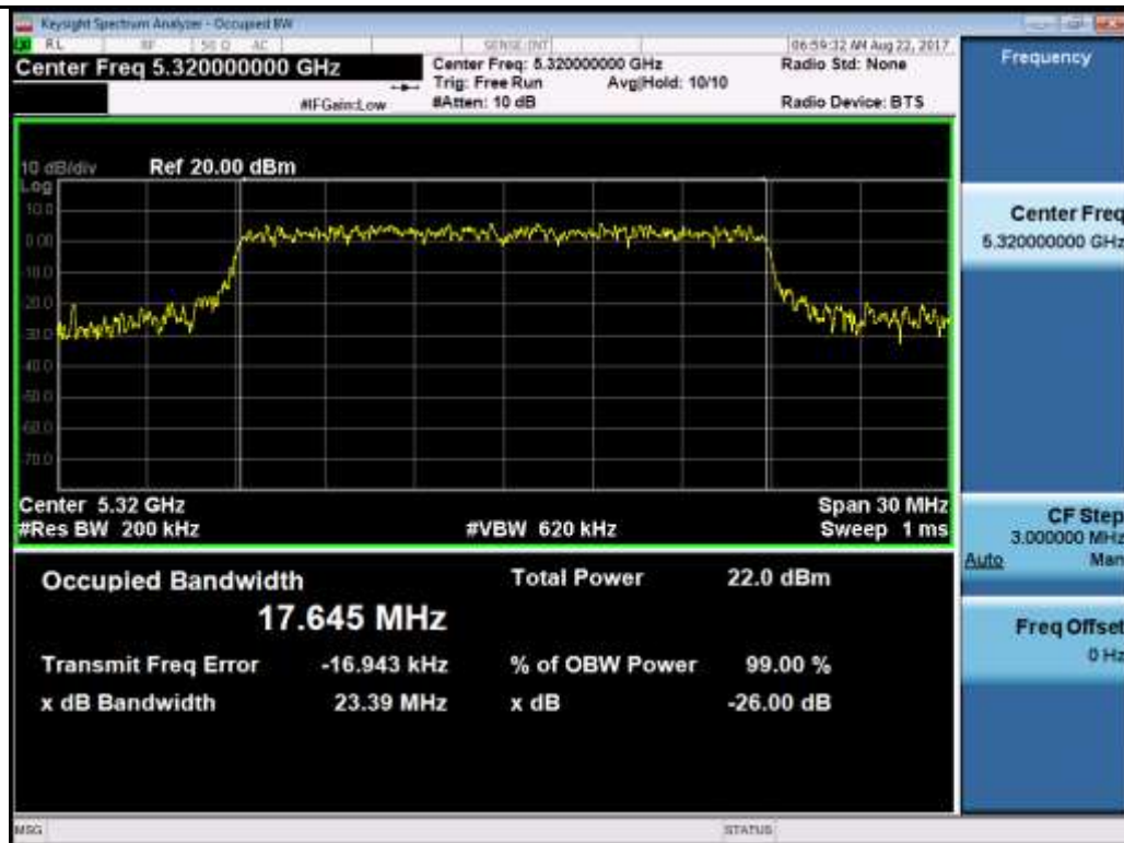
802.11n-HT20-5320MHz
