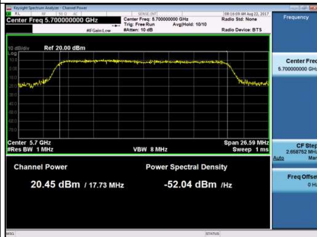
802.11n-HT20 5700M
