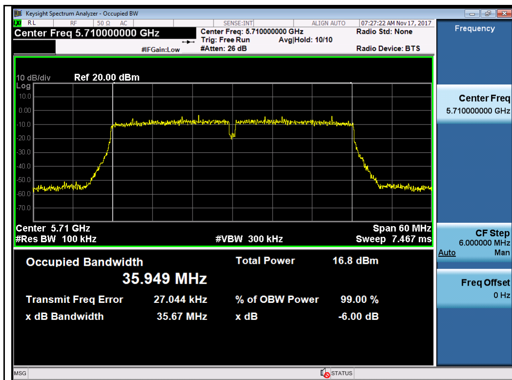
802.11n-HT40 5710MHz
