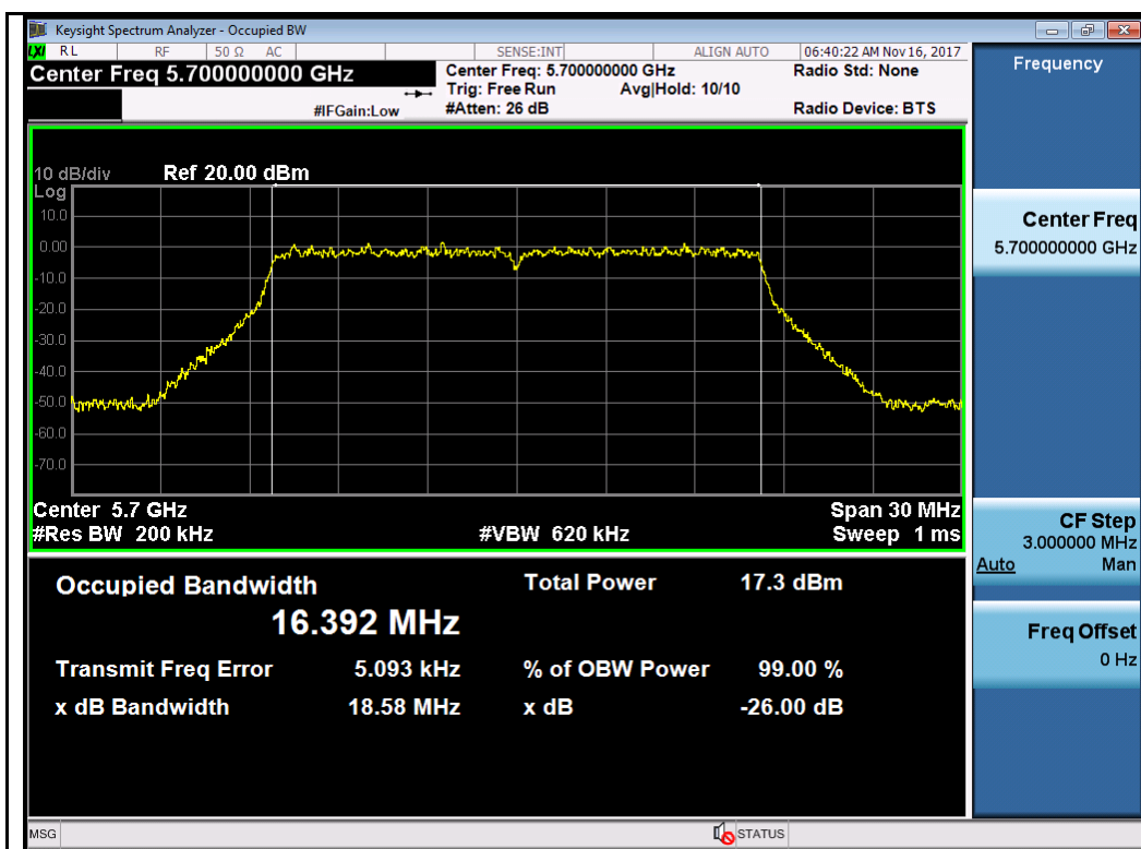
802.11a-5700MHz
