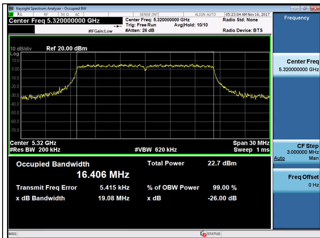
802.11a-5320MHz
