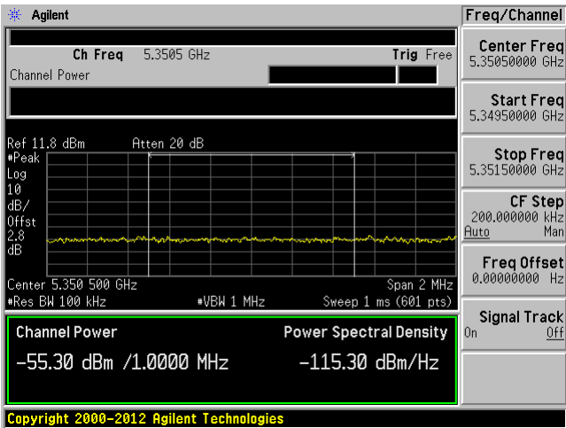
High Edge Chain 1
