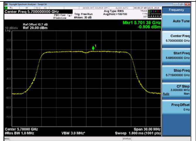
PSD-802.11n-20M-5700M-chain2
