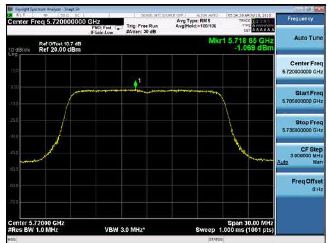
PSD-802.11n-20M-CROSS-5720M-chain4
