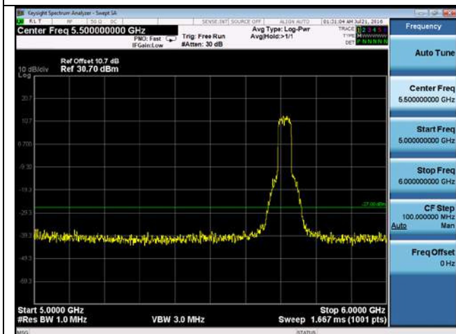
CUE-802.11n40-5710M -chain3(5GHz-6GHz)
