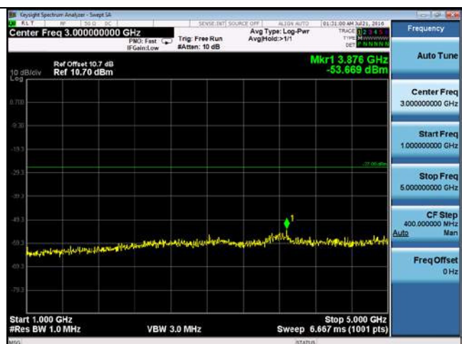
CUE-802.11n40-5710M -chain3(1GHz-5GHz)
