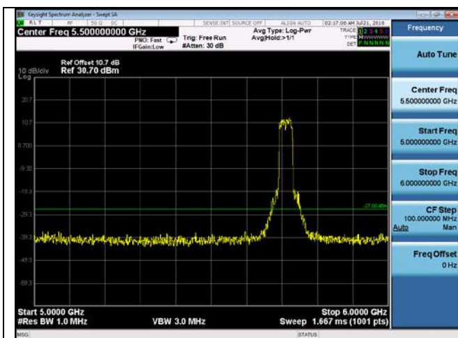
CUE-802.11n40-5710M -chain4 (5GHz-6GHz)
