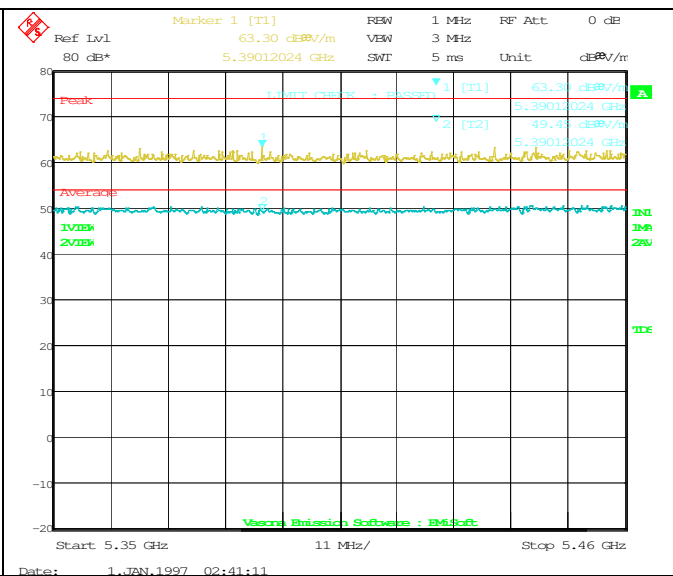
802.11n-HT20 5320M(5350-5460MHz)
