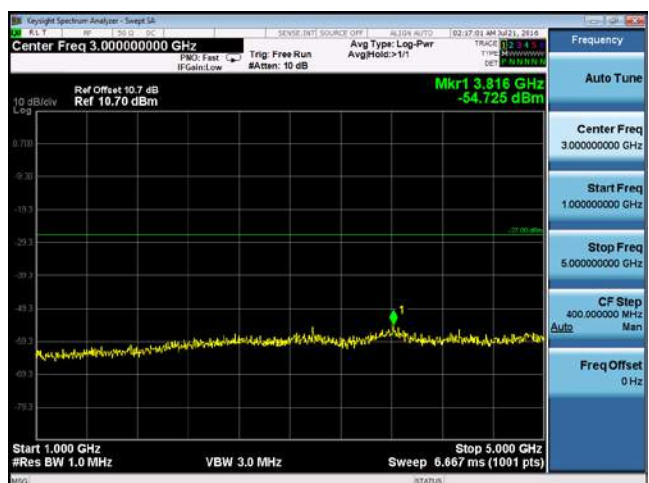
CUE-802.11n40-5710M -chain4(1GHz-5GHz)
