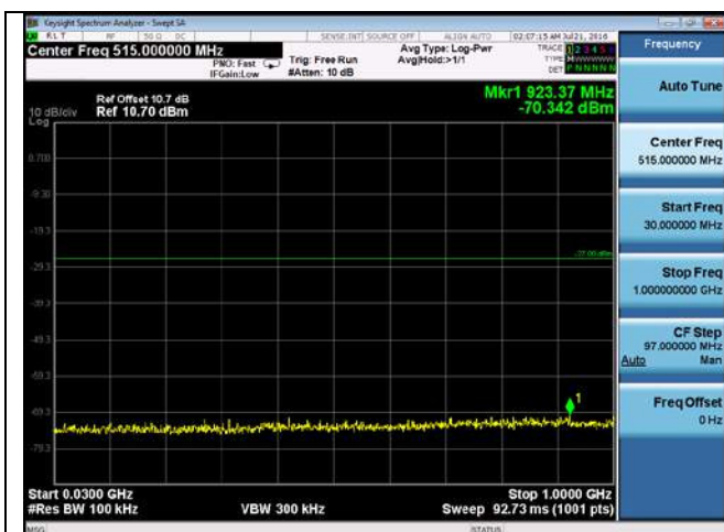
CUE-802.11n20-5720M -chain4(30MHz-1GHz)
