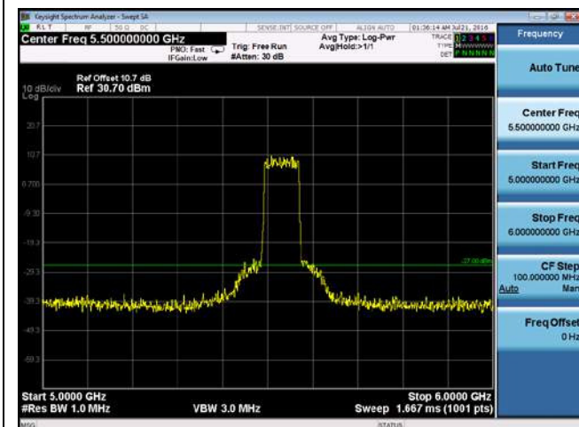
CUE-802.11ac-80-5530M -chain3(5GHz-6GHz)
