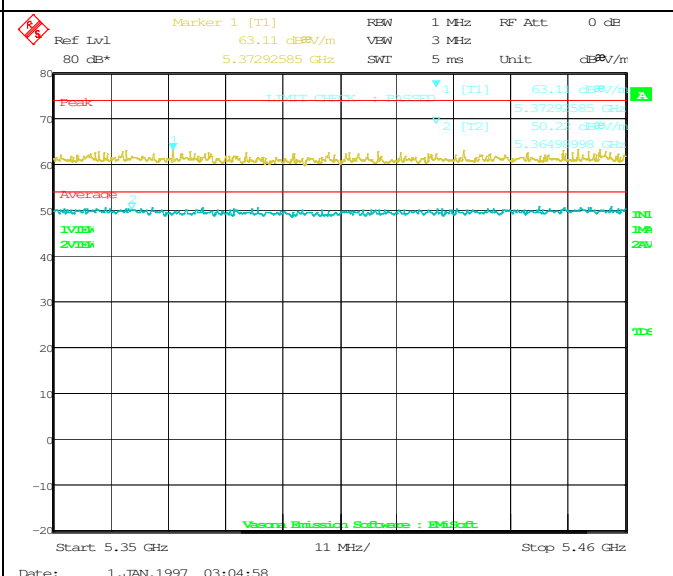
802.11ac 5290M(5350-5460MHz)
