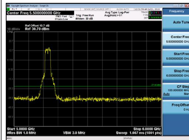
CUE-802.11n-40-5230M -chain2(5GHz-6GHz)
