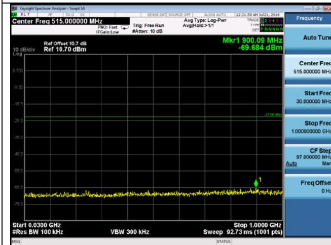
CUE-802.11n-40-5230M -chain2(30MHz-1GHz)
