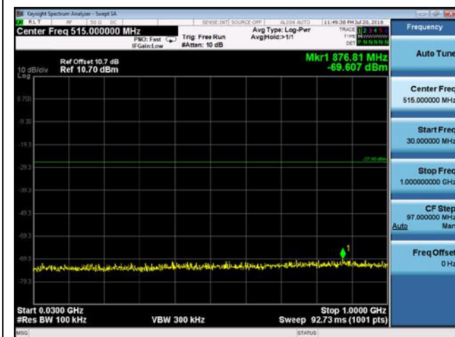
CUE-802.11n-20-5785M-chain1(30MHz-1GHz)
