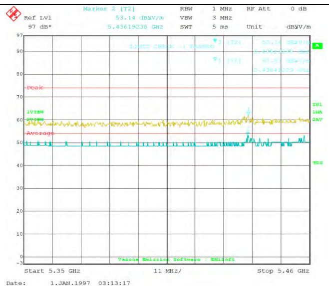
802.11ac 5530M(5350-5460MHz)
