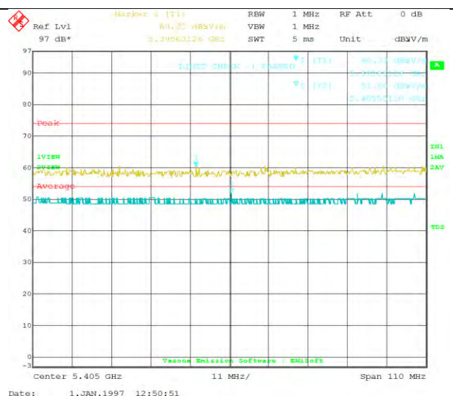
802.11n-HT20 5500M(5350-5460MHz)
