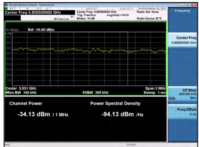
Band Edge -802.11n-20M-5825M-chain4
