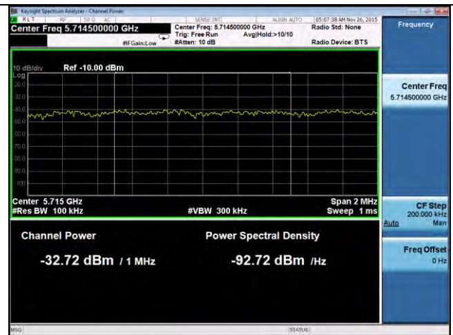
Band Edge -802.11n-40M-5755M-chain2
