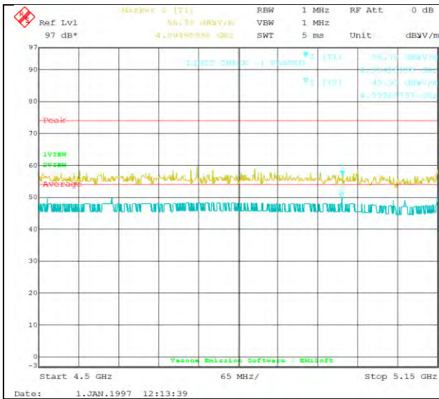
802.11a 5180M
