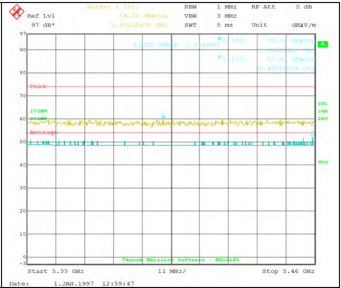
802.11n-HT40 5230M
