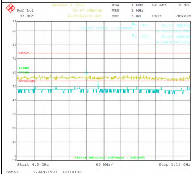
802.11n-HT20 5180M
