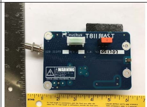
Bias-T Bottom View
