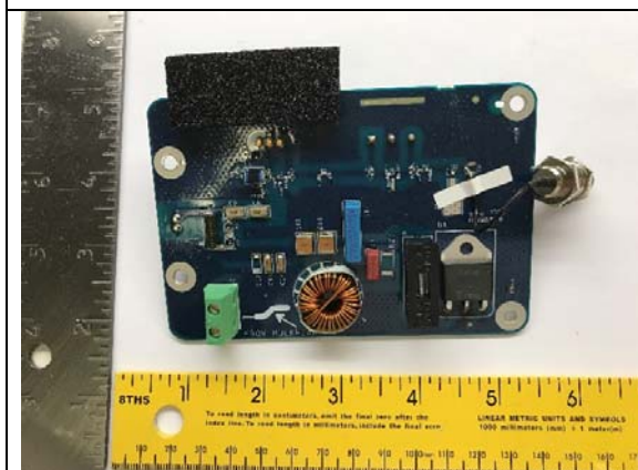
Bias-T Top View
