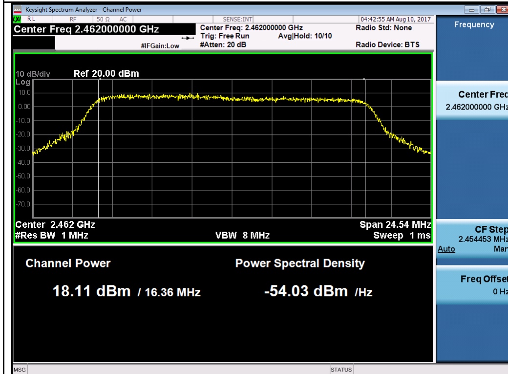
802.11g-2462MHz Chain 3
