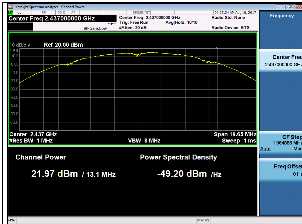
802.11b-2437MHz Chain 2
