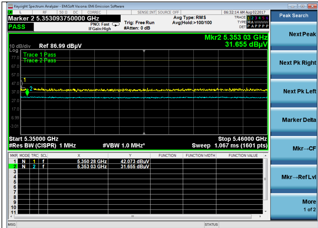
802.11a 5320M(5350-5460MHz)
