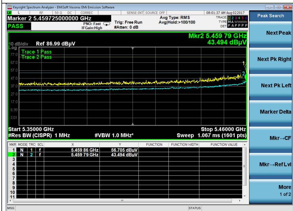
802.11a 5500M(5350-5460MHz)
