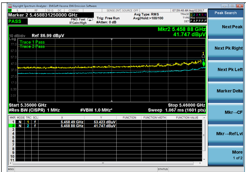
802.11a 5500M(5350-5460MHz)
